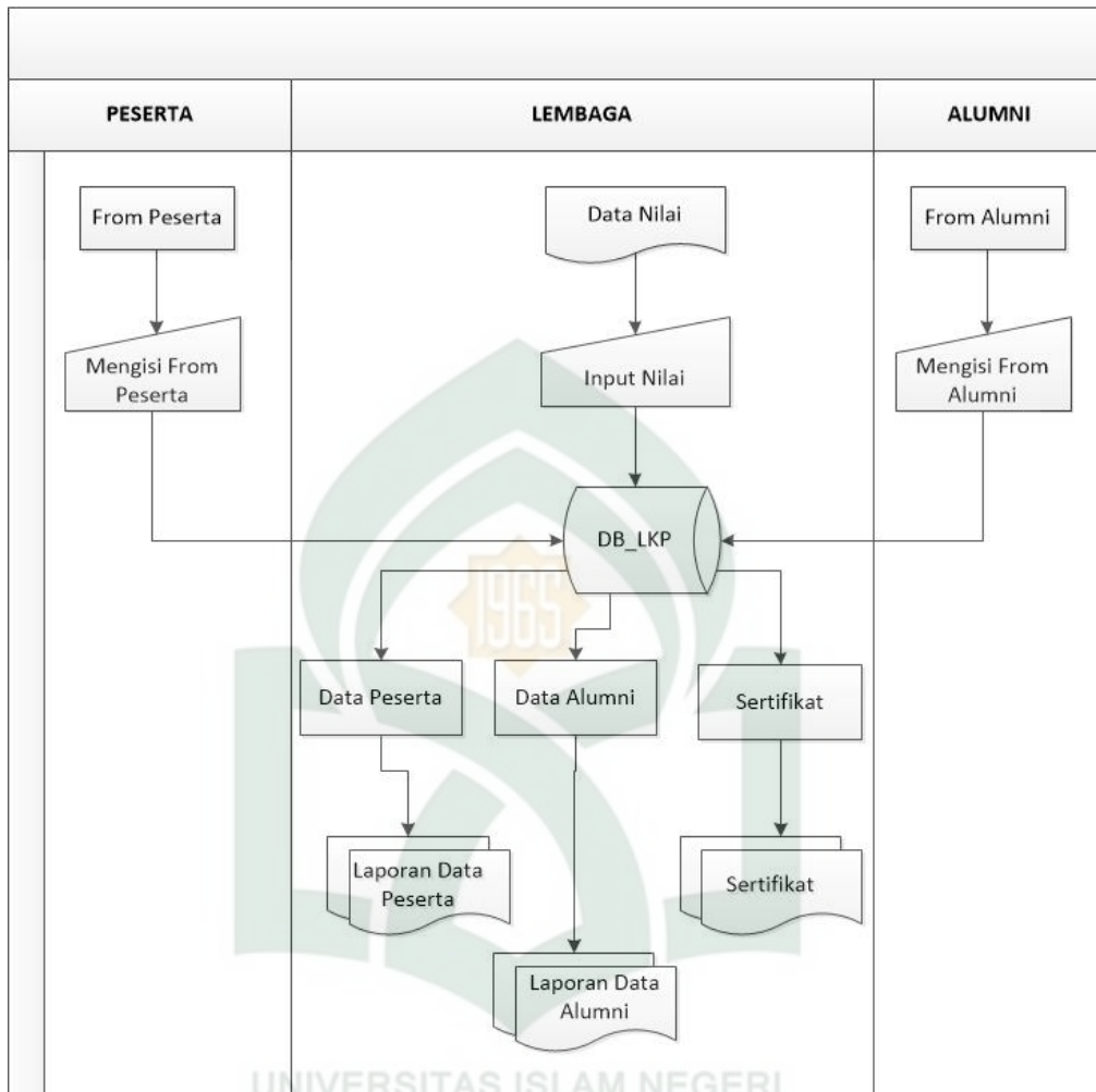
Gambar IV. 2. Flowmap sistem yang diusulkan
