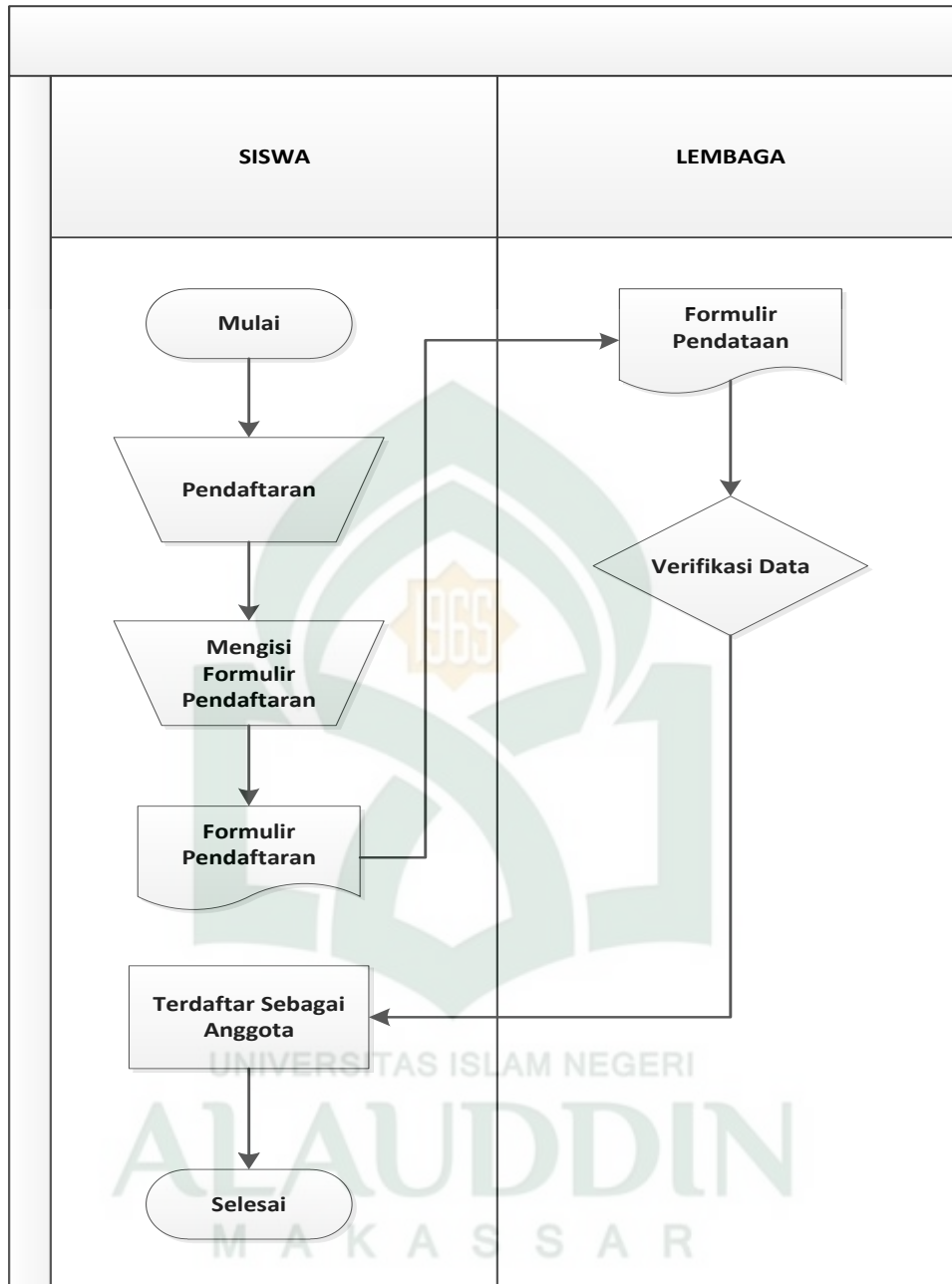
Gambar IV. 1. Flowmap Sistem yang sedang berjalan
