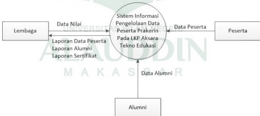
Gambar IV. 3. Diagram Konteks
