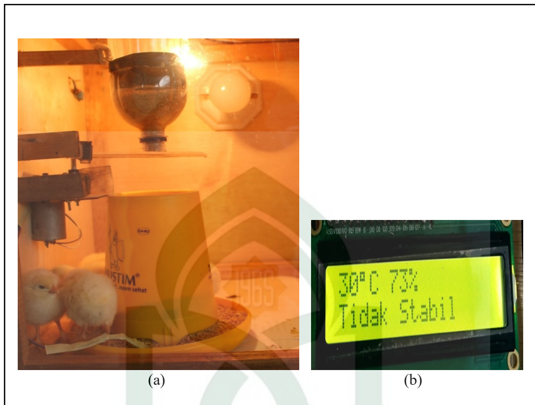
Gambar V.8. Pengujian Sensor DHT11 (Kondisi Tidak Stabil)
