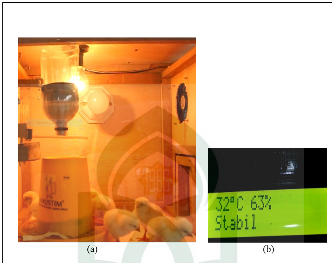
Gambar V.9. Pengujian Sensor DHT11 (Kondisi Stabil)
