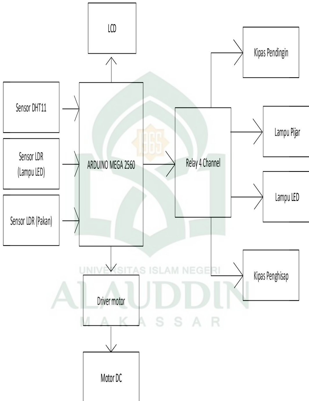
Gambar IV.1. Diagram Blok Sistem Alat
