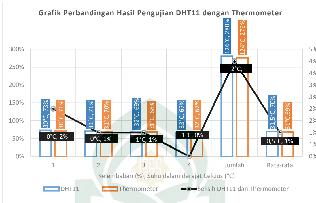
Gambar V. 5. Grafik Perbandingan Sensor DHT11 dan Thermometer
