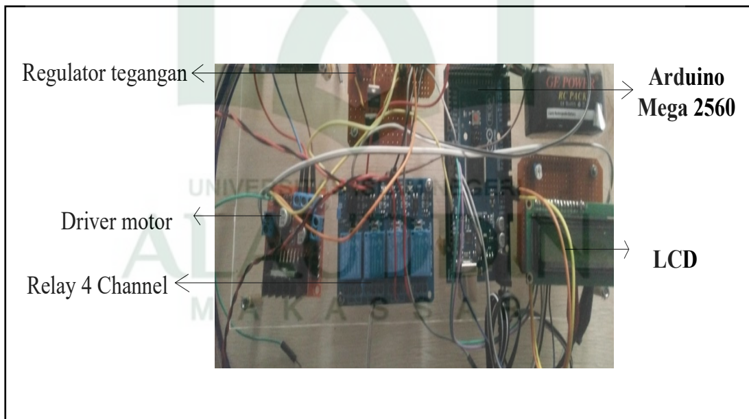
Gambar V.3. Rangkaian Sistem Elektronika
