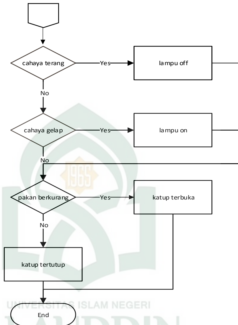
Gambar IV.11. Flowchart Sistem Alat
