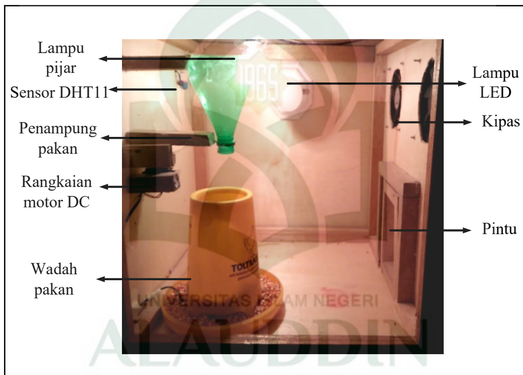
Gambar V.1. Prototype Kandang Tampak Depan
