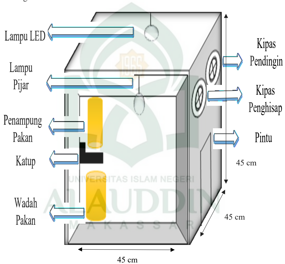
Gambar IV.3. Rangkaian Mekanik Prototype Kandang
