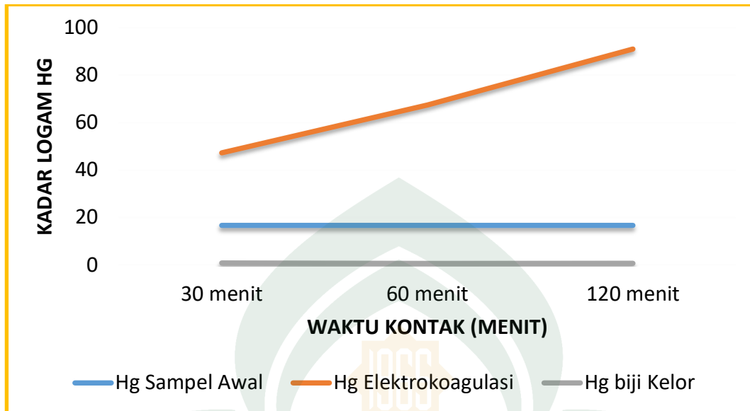
Grafik 4.12 : Pengaruh Elektrokoagulasi untuk tegangan 12 volt dan koagulan biji kelor terhadap Hg
