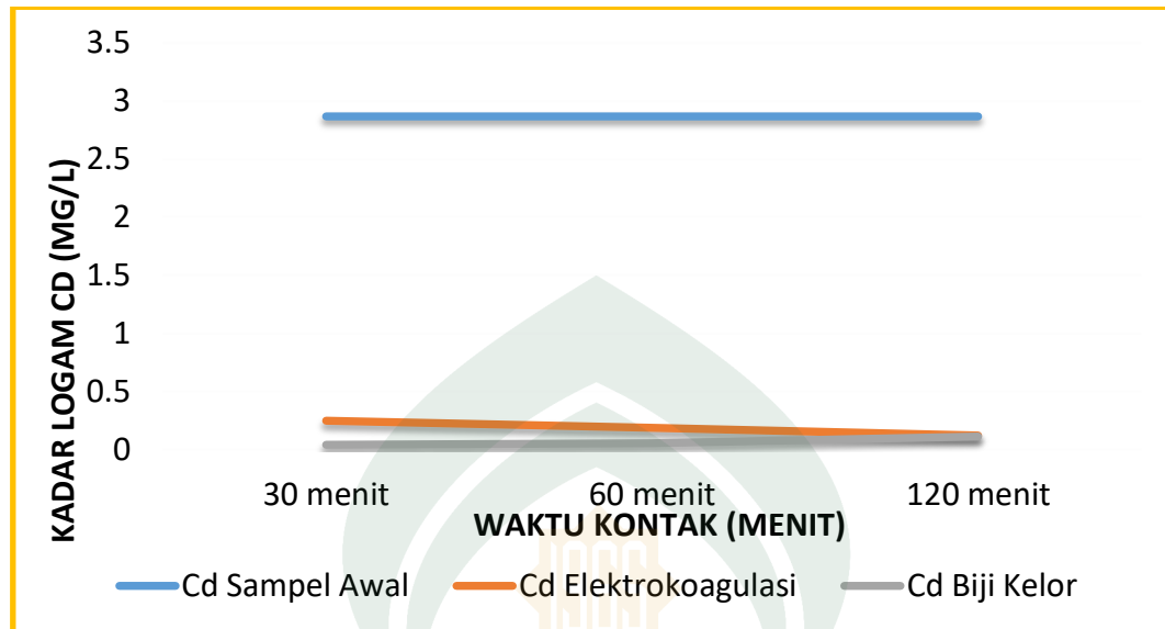
Grafik 4.18 : Pengaruh Elektrokoagulasi untuk tegangan 12 volt dan koagulan biji kelor terhadap Cd
