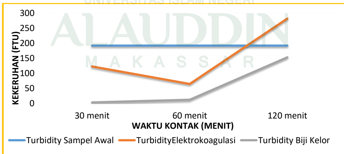
Grafik 4.4 : Pengaruh Elektrokoagulasi untuk tegangan 6 volt dan koagulan biji kelor terhadap kekeruhan ( turbidity )
