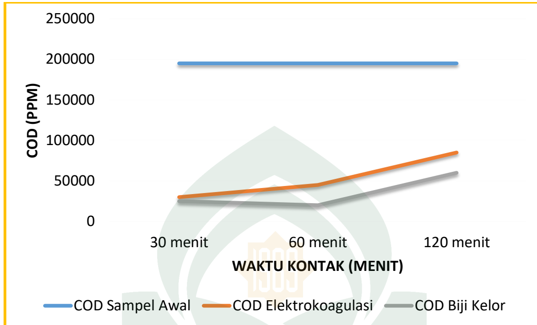
Grafik 4.8 : Pengaruh Elektrokoagulasi untuk tegangan 9 volt dan koagulan biji kelor terhadap COD
