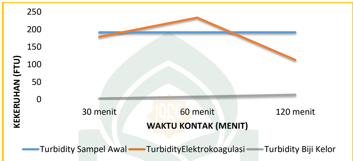
Grafik 4.6 : Pengaruh Elektrokoagulasi untuk tegangan 12 volt dan koagulan biji kelor terhadap kekeruhan ( turbidity )
