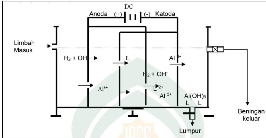
Gambar 2.2 Mekanisme reaksi yang terjadi pada proses
