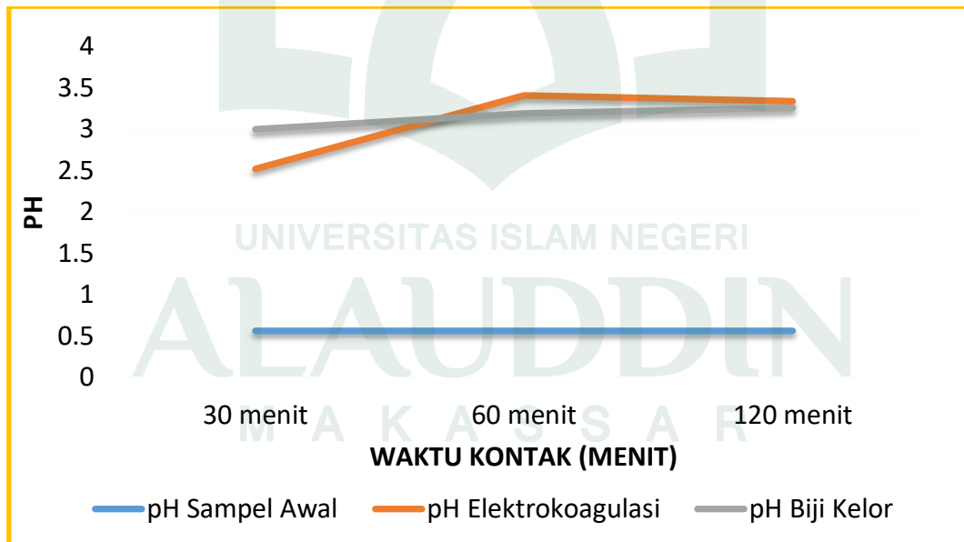
Grafik 4.3 : Pengaruh Elektrokoagulasi untuk tegangan 12 volt dan koagulan biji kelor terhadap pH
