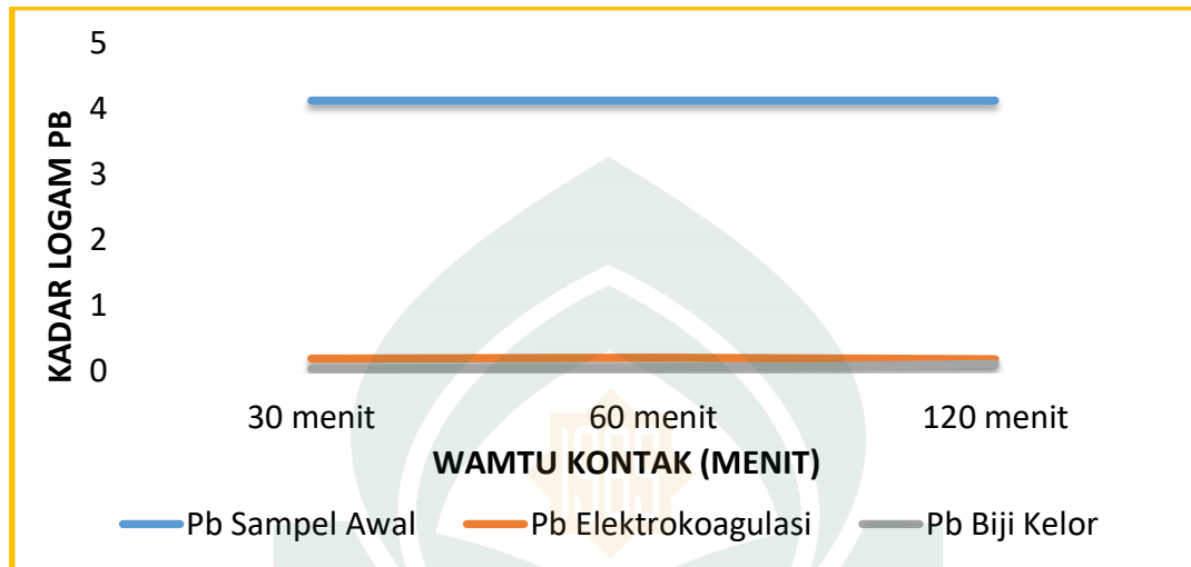
Grafik 4.15 : Pengaruh Elektrokoagulasi untuk tegangan 12 volt dan koagulan biji kelor terhadap Pb
