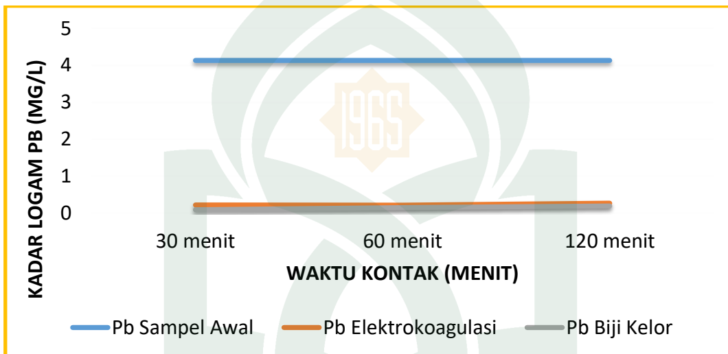
Grafik 4.13 : Pengaruh Elektrokoagulasi untuk tegangan 6 volt dan koagulan biji kelor terhadap Pb
