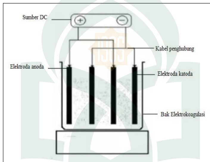
Gambar 2.3 Susunan Elektroda Paralel
