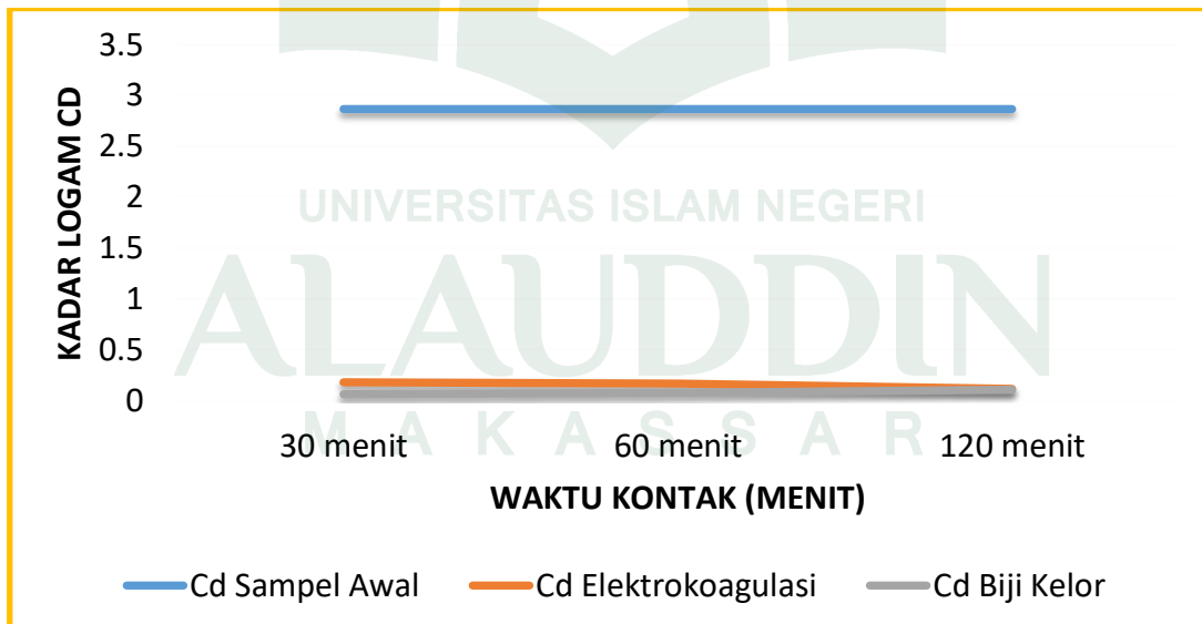
Grafik 4.17 : Pengaruh Elektrokoagulasi untuk tegangan 9 volt dan koagulan biji kelor terhadap Cd
