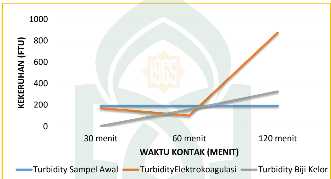
Grafik 4.4 : Pengaruh Elektrokoagulasi untuk tegangan 6 volt dan koagulan biji kelor terhadap kekeruhan ( turbidity )
