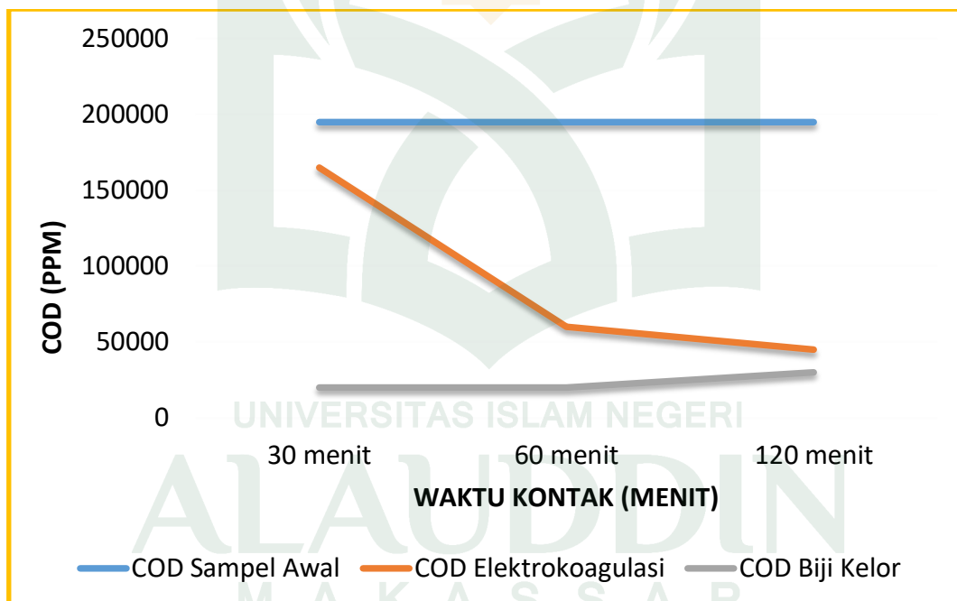
Grafik 4.7 : Pengaruh Elektrokoagulasi untuk tegangan 6 volt dan koagulan biji kelor terhadap COD
