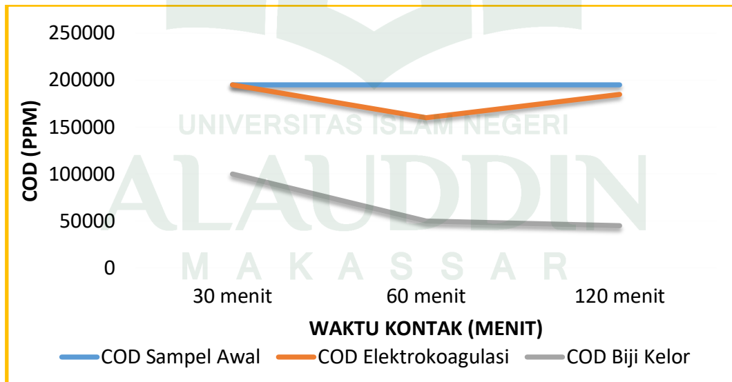
Grafik 4.9 : Pengaruh Elektrokoagulasi untuk tegangan 6 volt dan koagulan biji kelor terhadap COD
