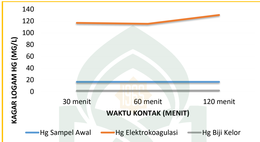
Grafik 4.10 : Pengaruh Elektrokoagulasi untuk tegangan 6 volt dan koagulan biji kelor terhadap Hg
