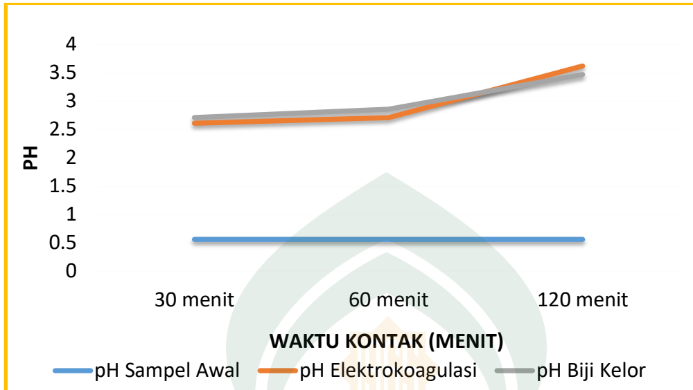
Grafik 4.2 : Pengaruh Elektrokoagulasi untuk tegangan 9 volt dan koagulan biji kelor terhadap pH
