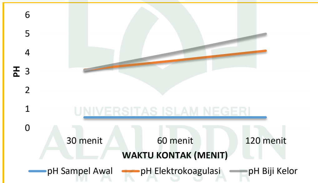
Grafik 4.1 : Pengaruh Elektrokoagulasi untuk tegangan 6 volt dan koagulan biji kelor terhadap pH
