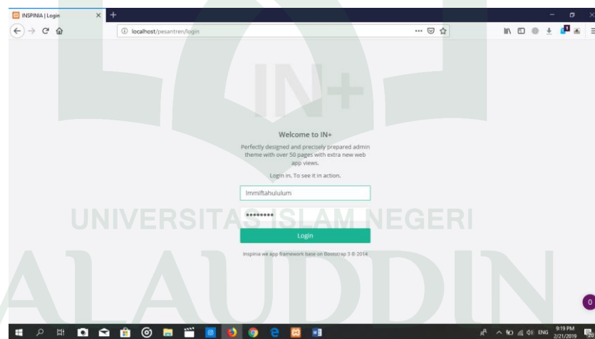
Gambar V.1 Halaman login
