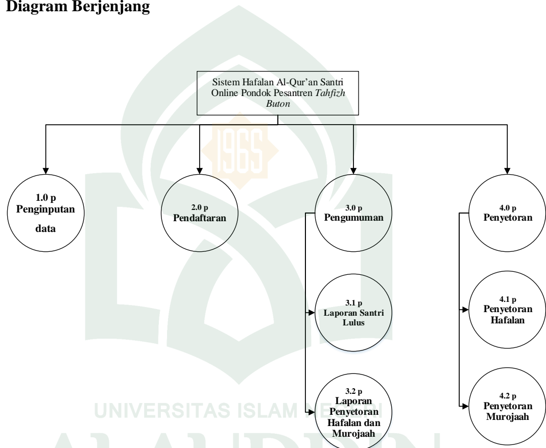
Gambar IV.3 Diagram Berjenjang
