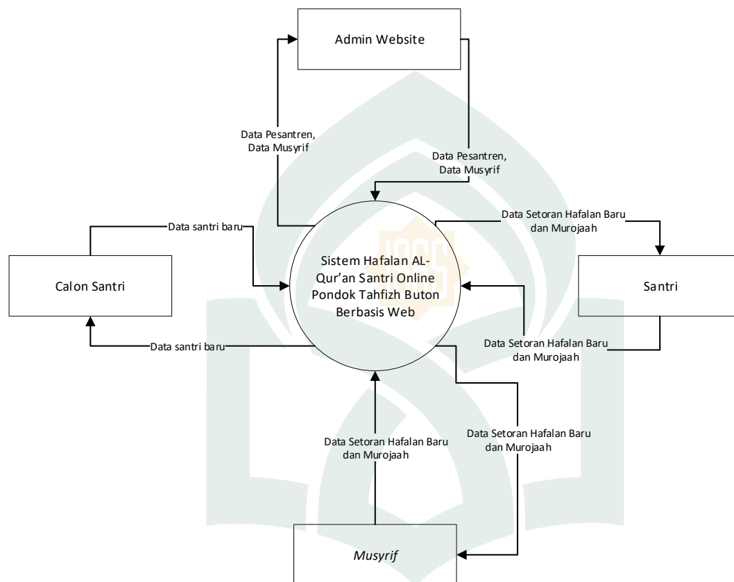
Gambar IV.4 Diagram Konteks
