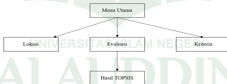
Gambar IV. 7 Struktur Navigasi
