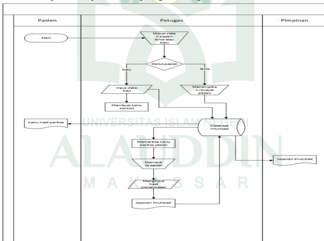
Gambar.IV 2 Flow Map Sistem yang diusulkan
