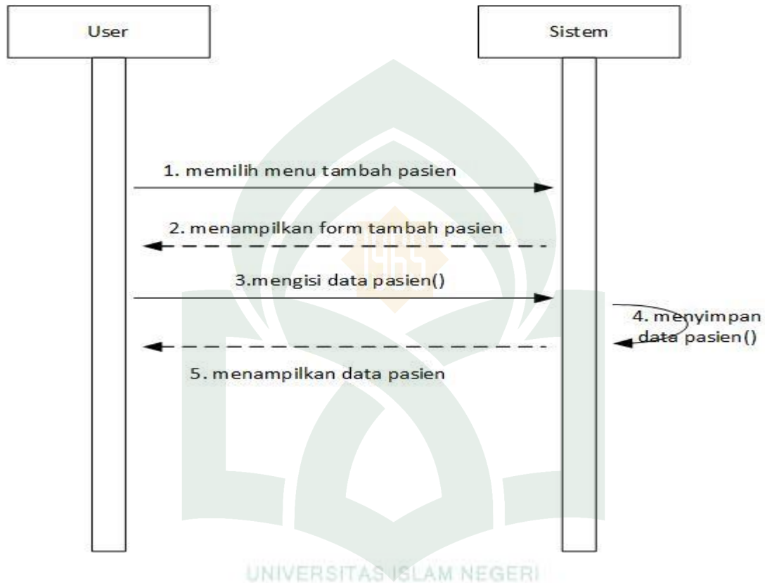
Gambar.IV 7 Sequence Sub Menu Tambah Pasien
