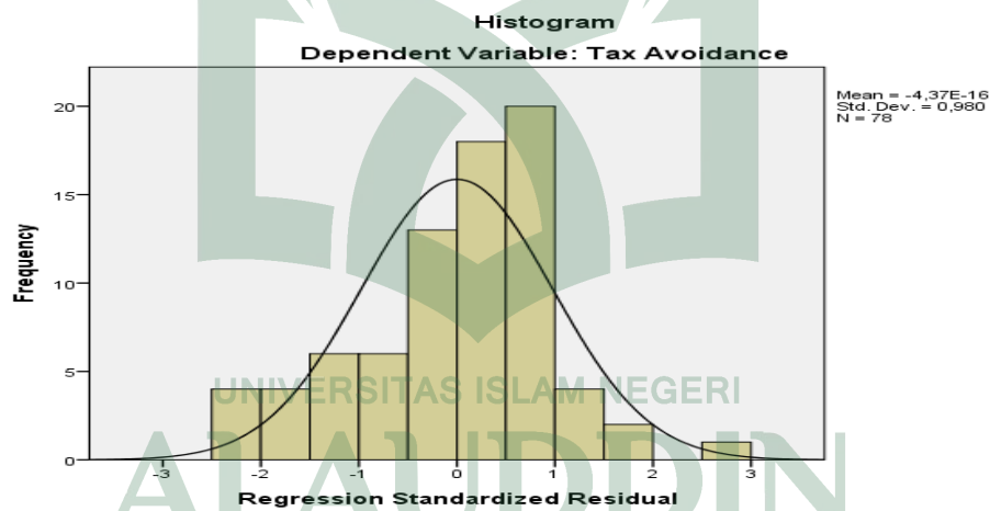
Gambar 4.1 Grafik Histogram
