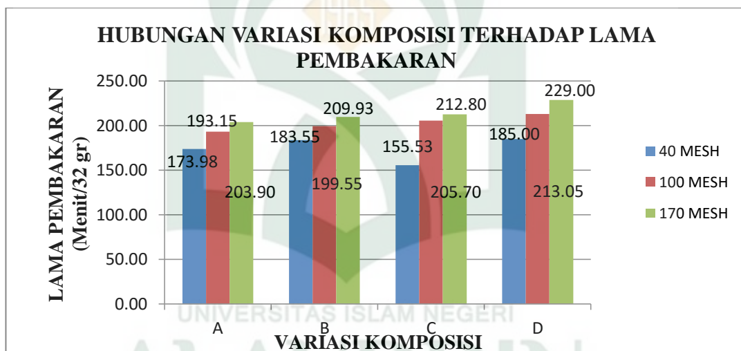
Grafik 4.3. Hubungan variasi komposisi terhadap lama pembakaran briket
