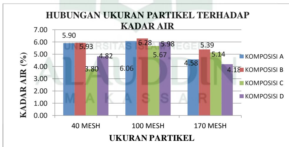
Grafik 4.5. Hubungan ukuran partikel terhadap kadar air briket
