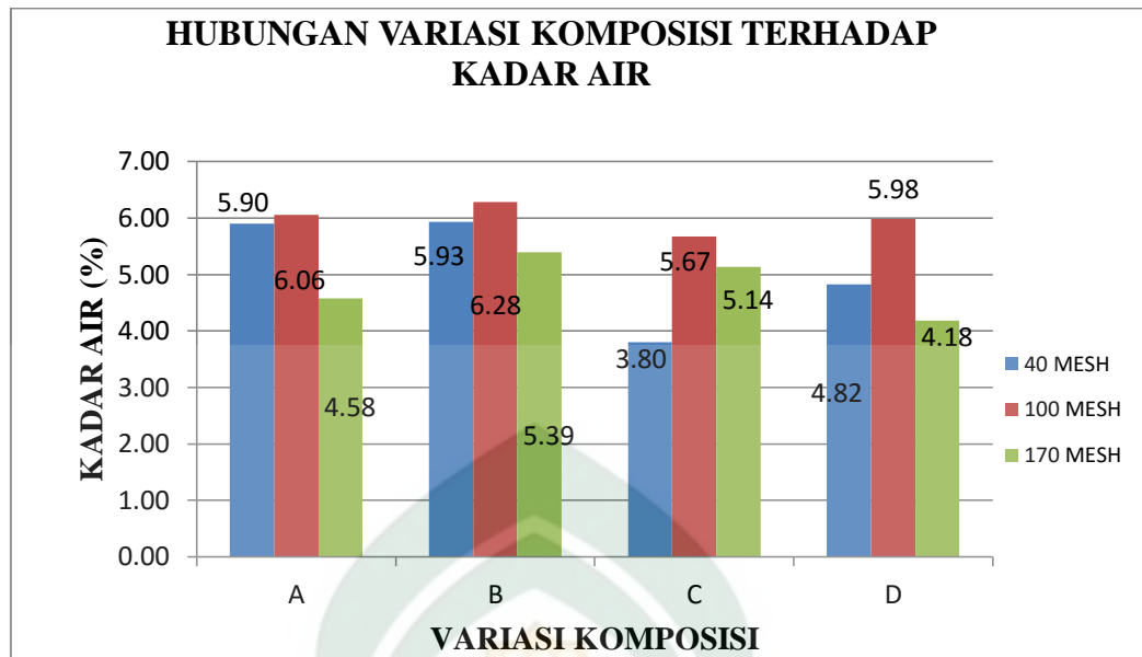
Grafik 4.2. Hubungan variasi komposisi terhadap kadar air briket
