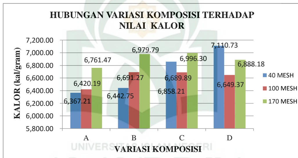
Grafik 4.1. Hubungan variasi komposisi terhadap nilai kalor
