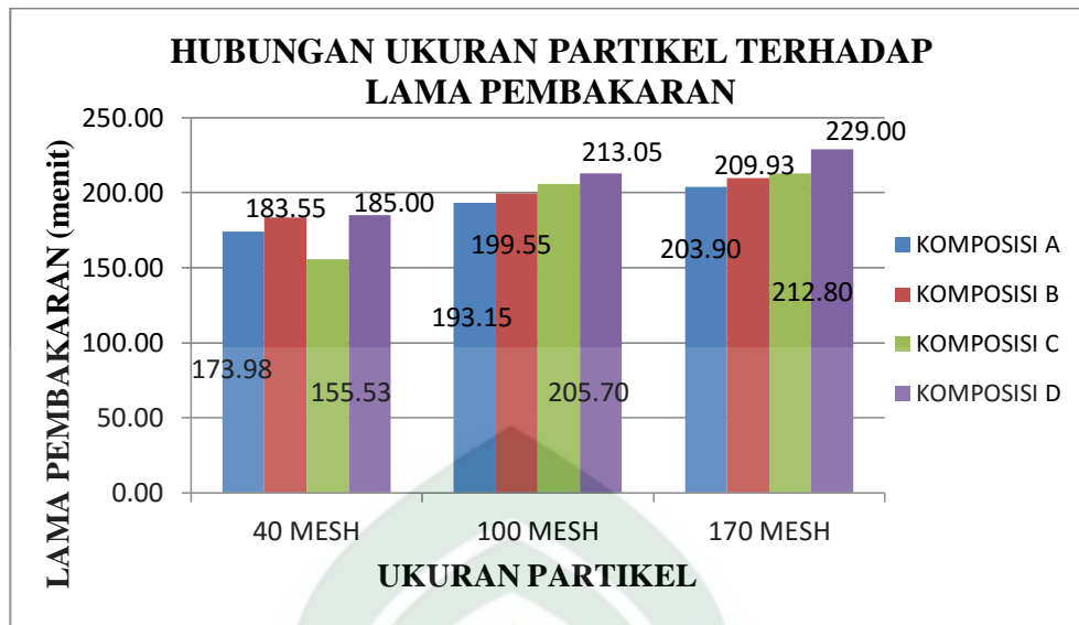
Grafik 4.6. Hubungan ukuran partikel terhadap lama pembakaran briket
