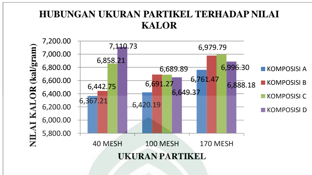
Grafik 4.4. Hubungan ukuran partikel terhadap nilai kalor briket
