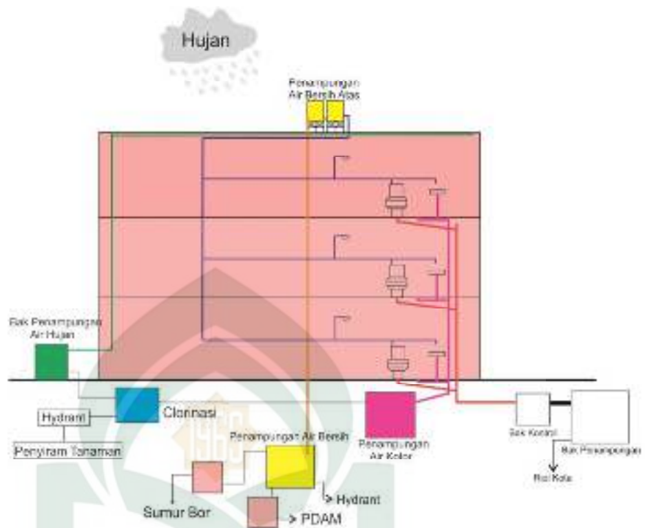
Gambar 3.20. Sistem air bersih dan air kotor Sumber : Olah Data, Tanggal 20 Desember 2017
