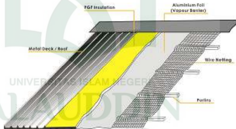
Gambar 3.11. insulator tahan panas
