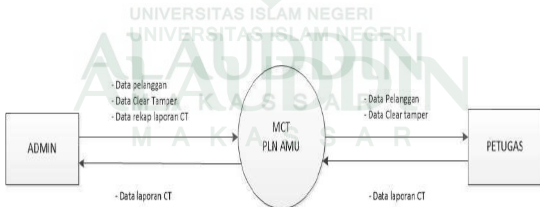
Gambar IV.6 Diagram Konteks
