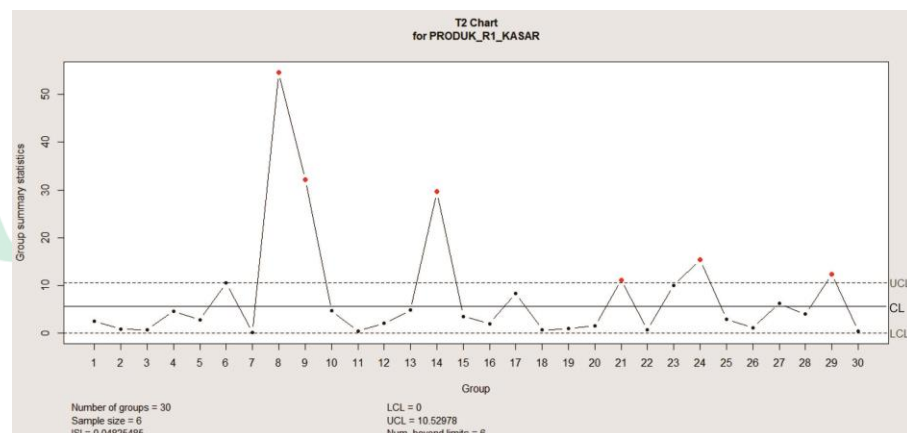
Gambar 4.21 Peta Kendali Multivariat T-Square Produk R1 Kasar
