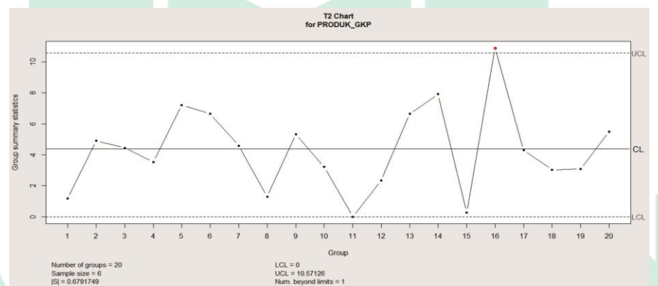
Gambar 4.29 Peta Kendali Multivariat T-Square Produk GKP Revisi 2
