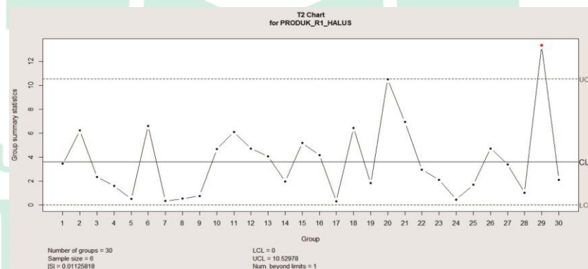
Gambar 4.24 Peta Kendali Multivariat T-Square Produk R1 Halus
