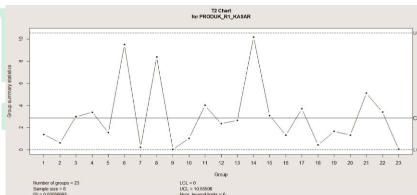
Gambar 4.23 Peta Kendali Multivariat T-Square Produk R1 Kasar Revisi 2
