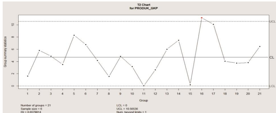
Gambar 4.28 Peta Kendali Multivariat T-Square Produk GKP Revisi 1
