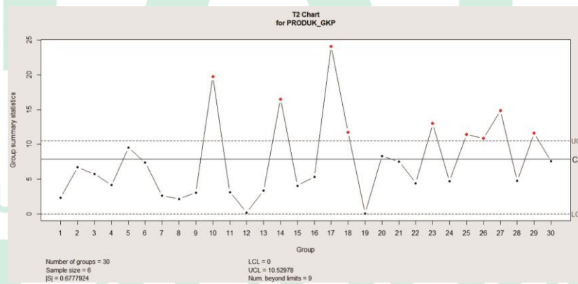
Gambar 4.27 Peta Kendali Multivariat T-Square Produk GKP
