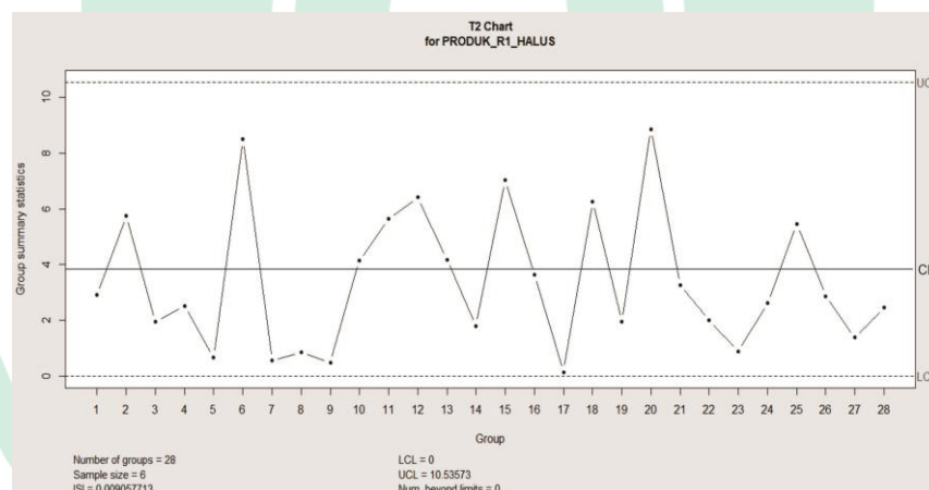
Gambar 4.26 Peta Kendali Multivariat T-Square Produk R1 Halus Revisi 2
