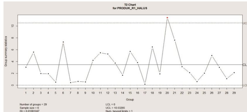
Gambar 4.25 Peta Kendali Multivariat T-Square Produk R1 Halus Revisi 1
