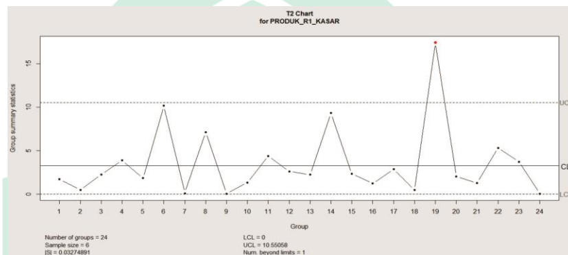
Gambar 4.22 Peta Kendali Multivariat T-Square Produk R1 Kasar Revisi 1
