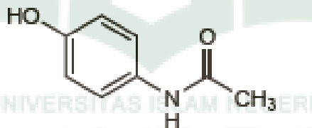
Gambar 7. Rumus Struktur Paracetamol
