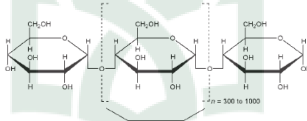
Gambar 5. Rumus Struktur Amilosa
