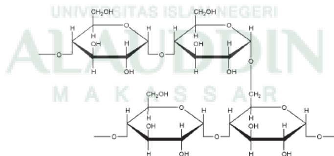
Gambar 6. Rumus Struktur Amilopektin (Sumber: Rowe, et al. 2009: 685).
