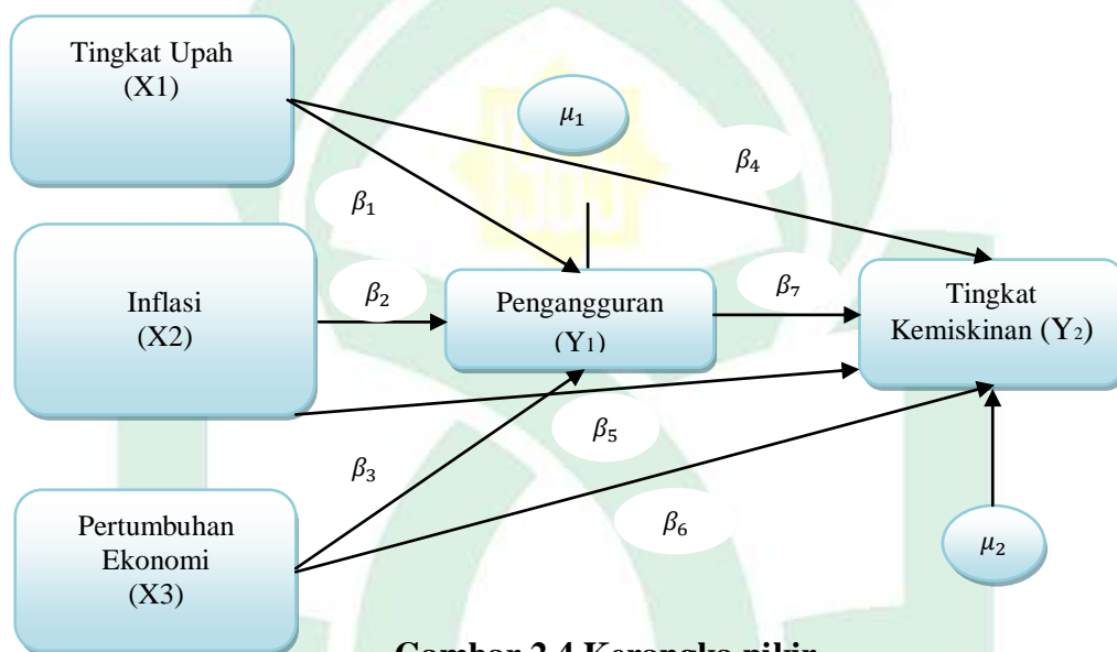
Gambar 2.4 Kerangka pikir
