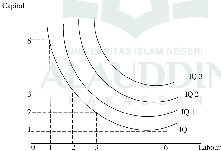
Gambar 1.1 Kurva Produksi
