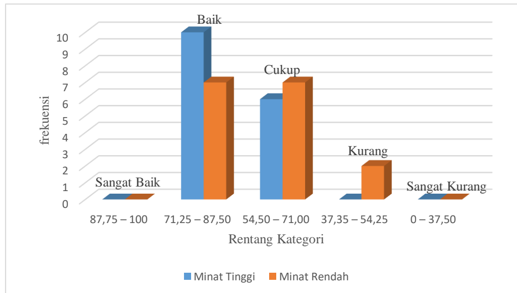
Grafik 4.2: Histogram Kategori Hasil Belajar Fisika Minat Tinggi dan Minat Rendah
