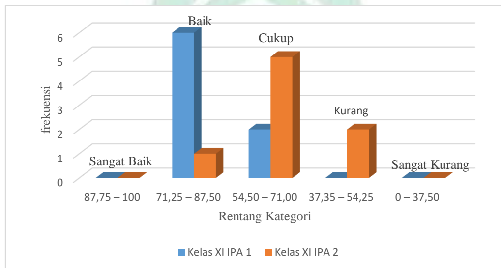
Grafik 4.4: Histogram Kategori Hasil Belajar Fisika Kelas Eksperimen I Dan Kelas Eksperimen II
