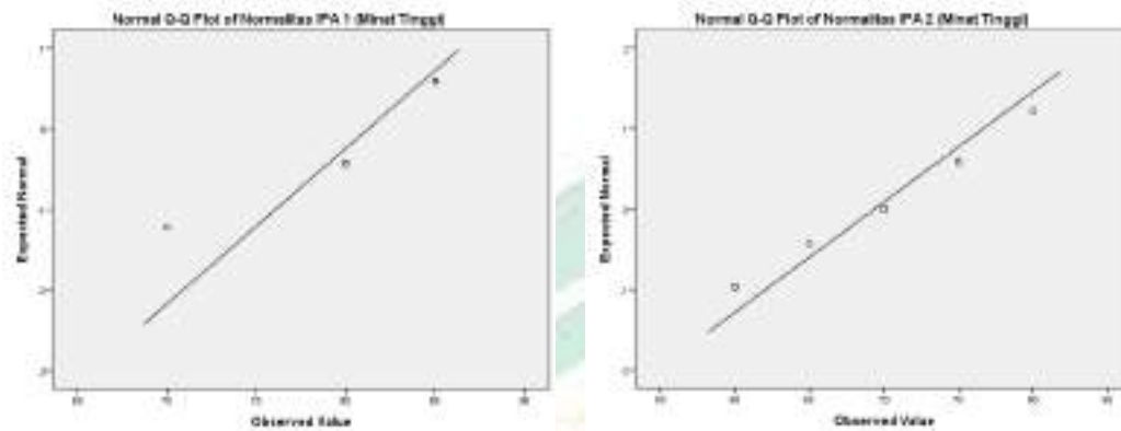
Gambar 4.4: Grafik Distribusi Normal Hasil Belajar Fisika Peserta Didik Minat Tinggi Kelas Eksperimen I dan Kelas Eksperimen II
