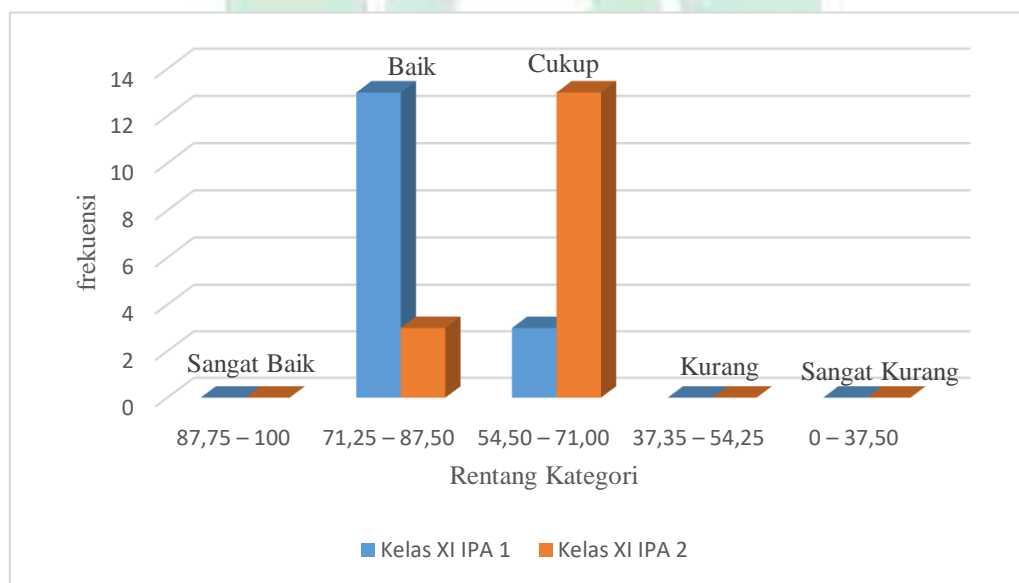
Grafik 4.1: Histogram Kategori Hasil Belajar Fisika Kelas Eksperimen I Dan Kelas Eksperimen II
