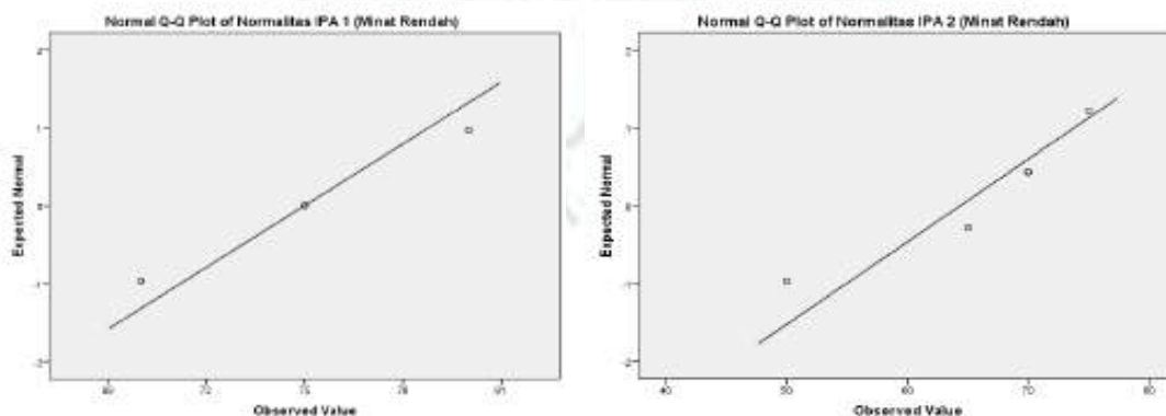
Gambar 4.5: Grafik Distribusi Normal Hasil Belajar Fisika Peserta Didik Minat Rendah Kelas Eksperimen I dan Kelas Eksperimen II
