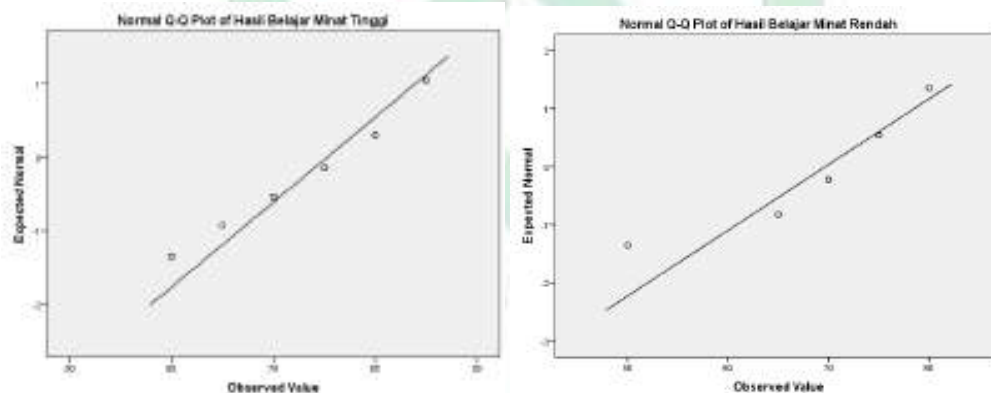
Gambar 4.2: Grafik Distribusi Normal Hasil Belajar Fisika Peserta Didik Minat Belajar Tinggi dan Minat Rendah
