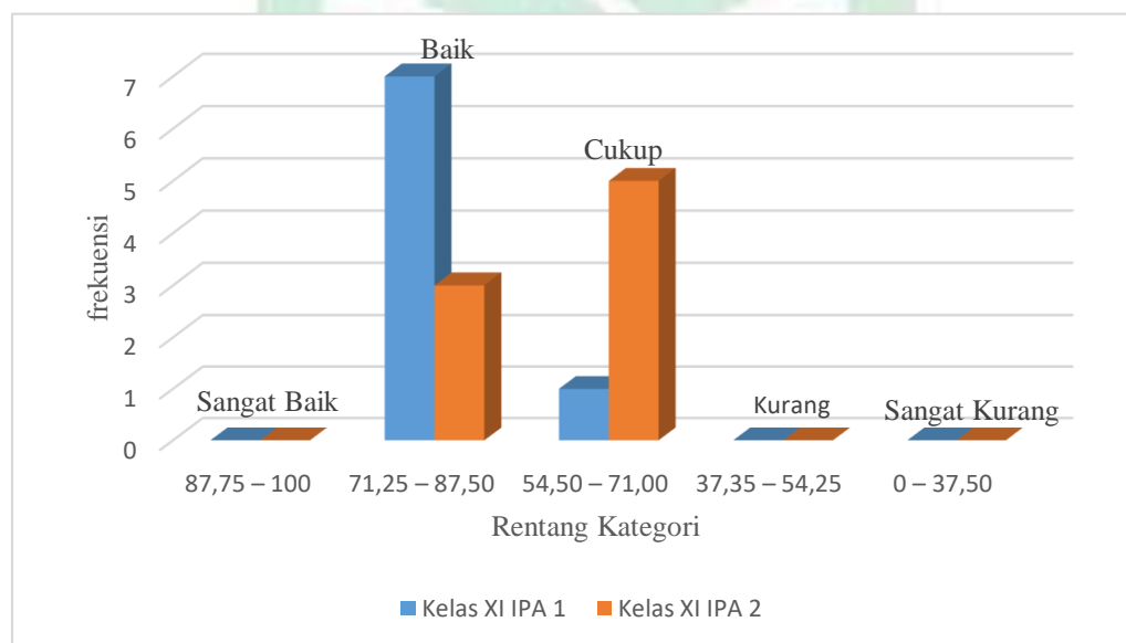
Grafik 4.3: Histogram Kategori Hasil Belajar Fisika Kelas Eksperimen I Dan Kelas Eksperimen II
