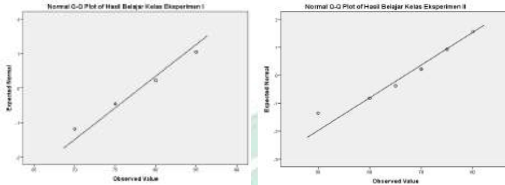
Gambar 4.1: Grafik Distribusi Normal Hasil Belajar Fisika Peserta Didik Kelas Eksperimen I dan Kelas Eksperimen II
