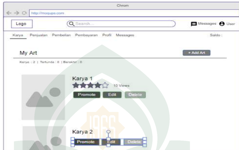
Gambar IV.13. Antarmuka Dashboard
