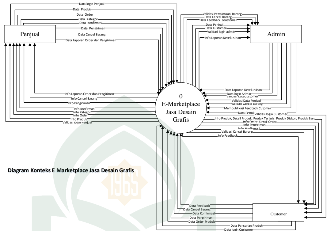
Gambar IV.4. Diagram Konteks
