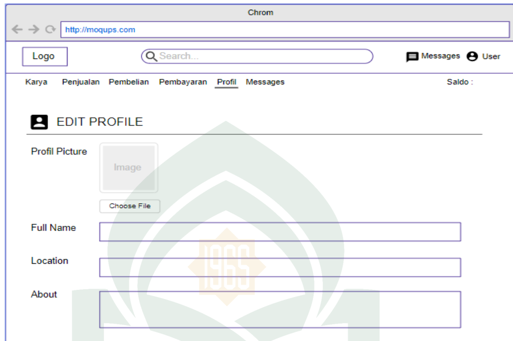
Gambar IV.17. Antarmuka Profile
