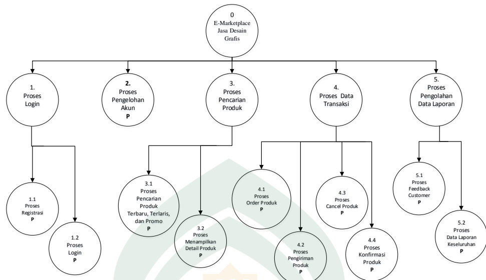
Gambar IV.3. Diagram Berjenjang
