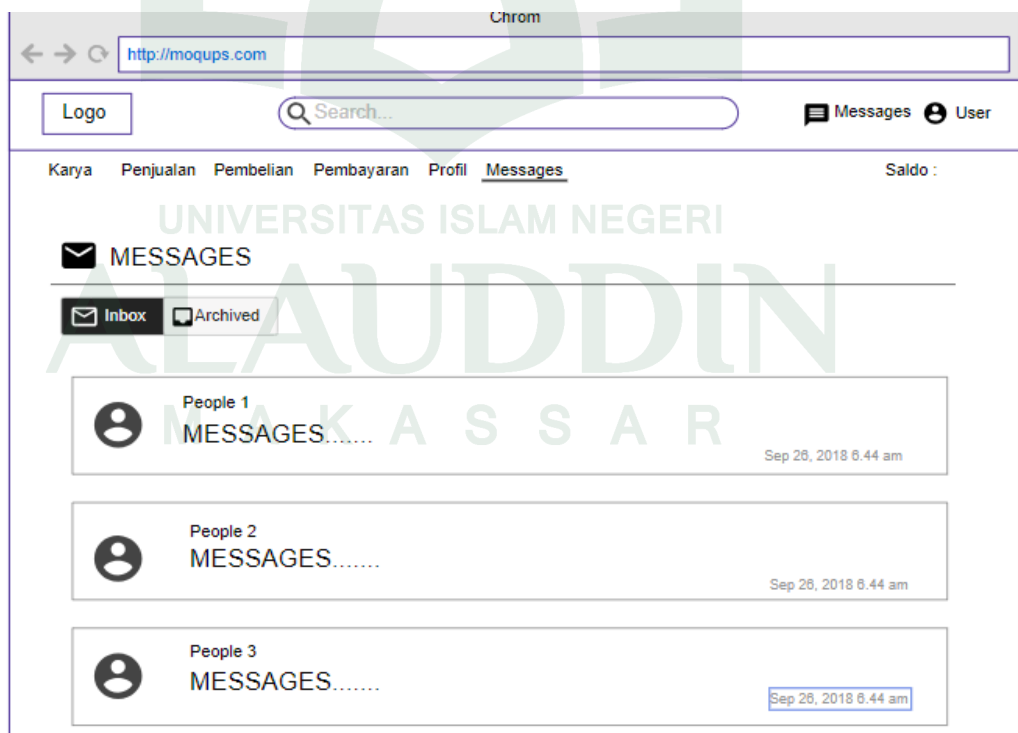
Gambar IV.18. Antarmuka Messages
