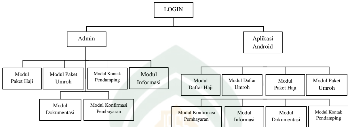
Gambar III.2 Hirarki pengujian integrasi
