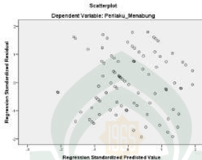
Gambar 4.3 Grafik Scatterplot
