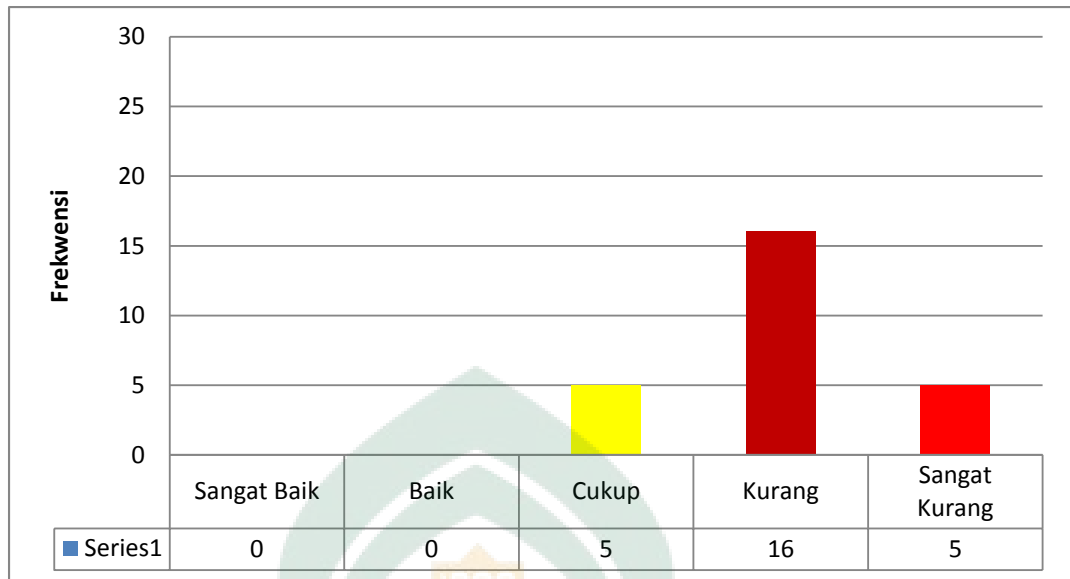
Grafik 4.1. Histogram Kategori Keterampilan Proses sains sebelum diterapkan Pembelajaran berbasis alat peraga
