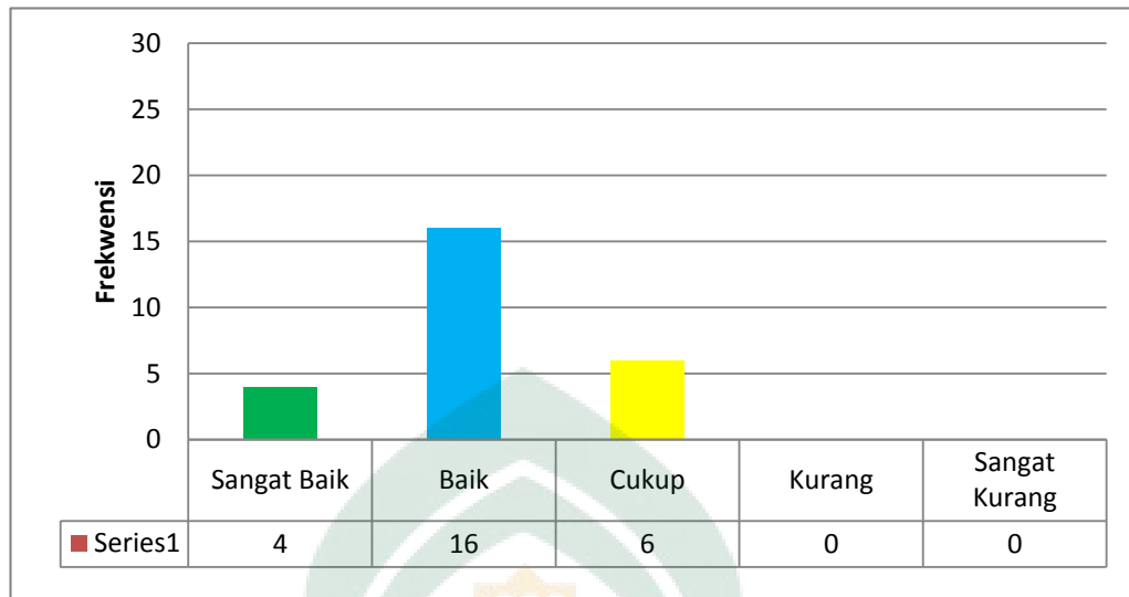
Grafik 4.2. Histogram Kategori Keterampilan proses sains setelah diterapkan Pembelajaran berbasis media alat peraga
