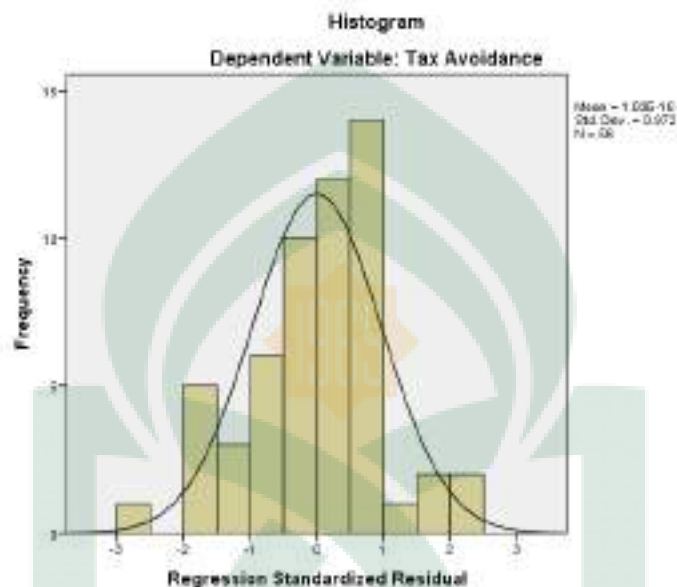
Gambar 4.1 Hasil Uji Normalitas – Grafik Histogram
