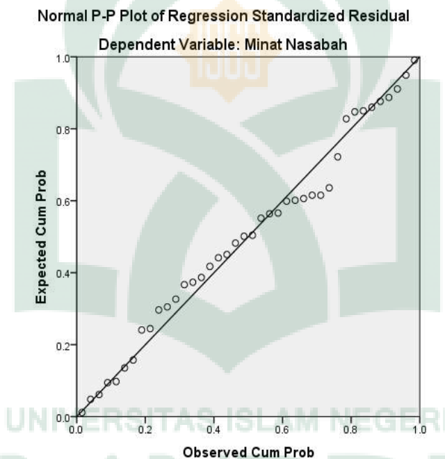
Gambar 4.1 Normalitas Data (P-P Plot)
