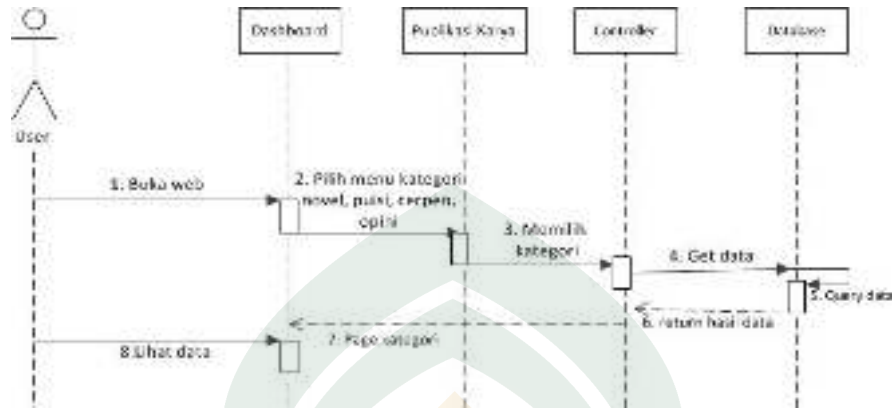
Gambar IV.8 Sequence diagram publikasi karya
