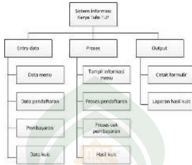
Gambar IV.12. Diagram HIPO
