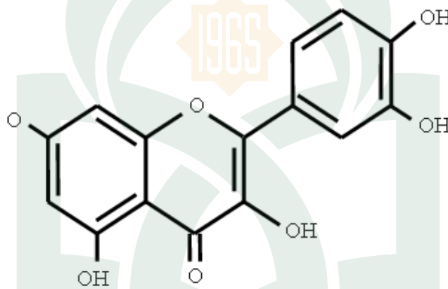
Gambar. II.3 kerangka dasar dari Flavonoid C_6-C_3-C_6
