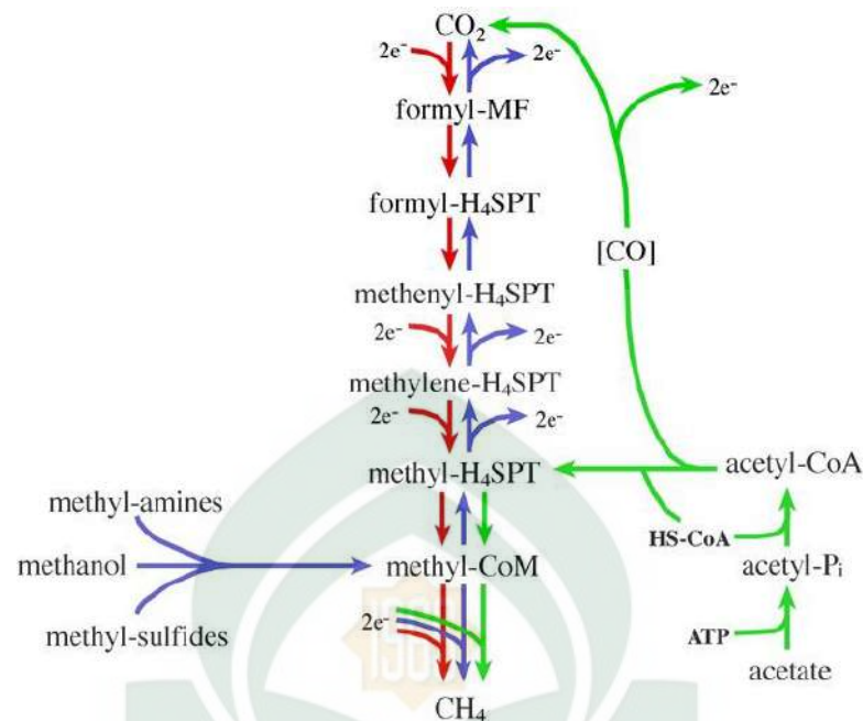
Gambar 4.2. Jalur Metanogenesis
