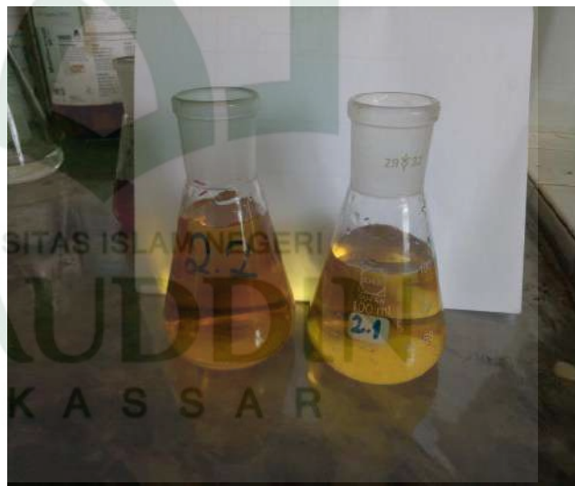
Proses Titrasi
