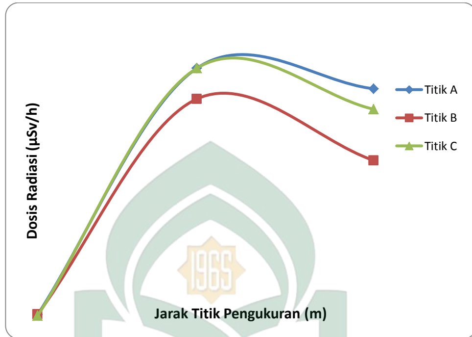
Gambar 4.2 grafik nilai dosis radiasi yang diterima dinding belakang pesawat pada berbagai ketinggian.
