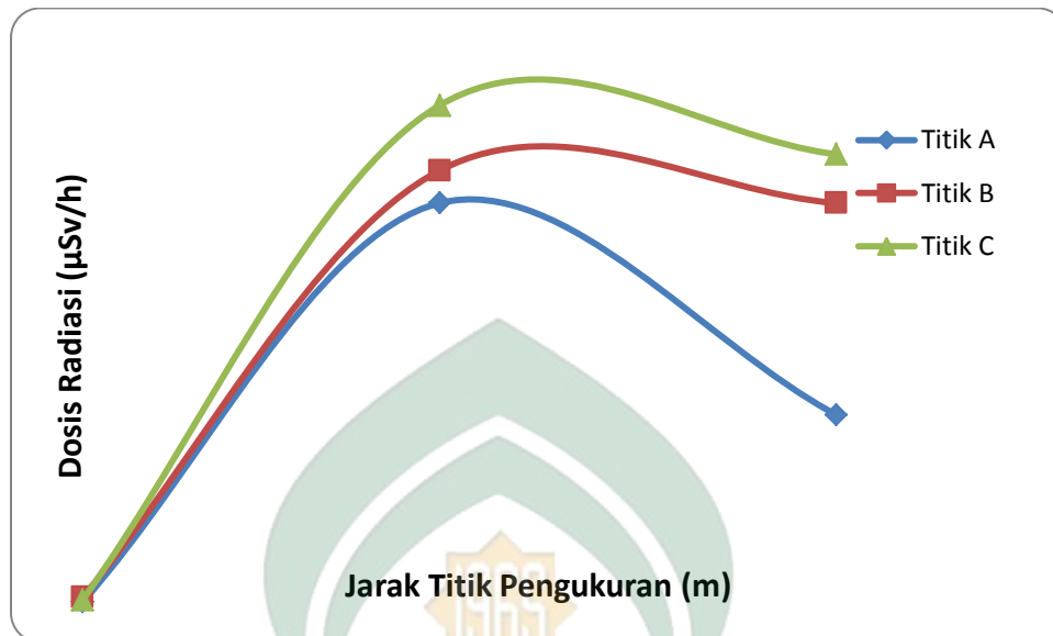
Gambar 4.4 grafik nilai dosis radiasi yang diterima dinding kanan pesawat pada berbagai ketinggian.
