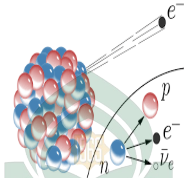
Gambar 2.2 Peluruhan Beta Sumber: Wikipedia.com 2015
