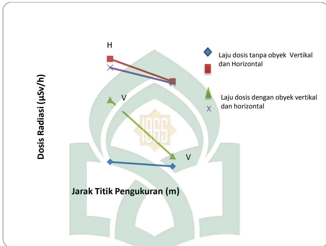
Gambar 4.8 grafik hubungan laju dosis radiasi dengan jarak titik pengukuran vertikal dan horizontal belakang pesawat.
