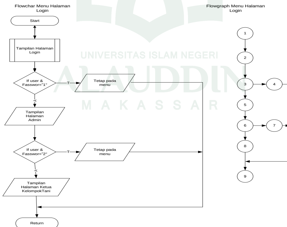
Gambar V.21. Flowchart dan Flowgraph Halaman Login.
