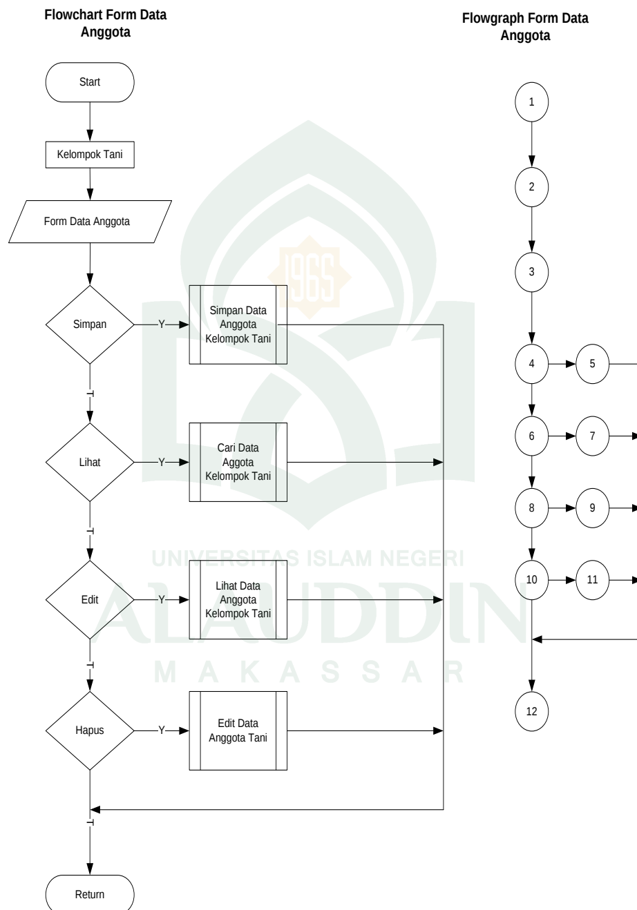
Gambar V.25. Flowchart dan Flowgraph Menu Data Anggota
