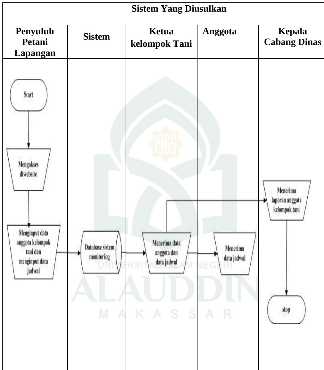
Gambar IV.2. Flow Map Diagram pada Sistem yang Diusulkan
