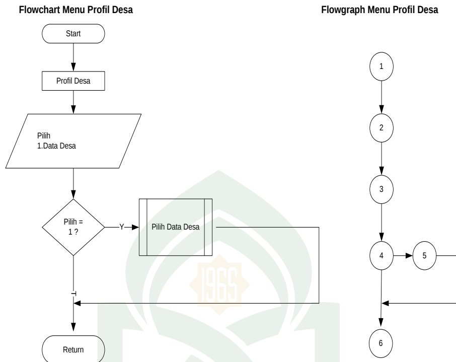
Gambar V.22. Flowchart dan Flowgraph Menu Data Profil Desa
