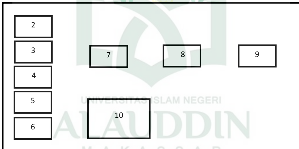
Gambar IV.10 Antarmuka Dasbor
