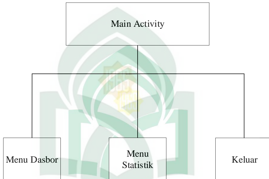
Gambar IV. 7 Struktur Navigasi
