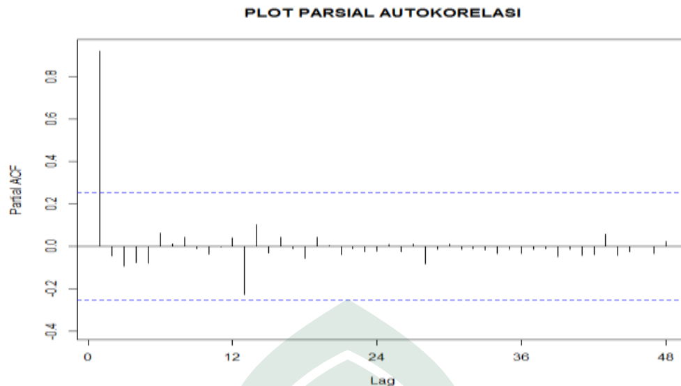
Gambar 4.5 Fungsi parsial autokorelasi (PACF) data asli jumlah pemilik kendaraan yang melakukan tunggakan Tahun 2014 sampai Tahun 2018
