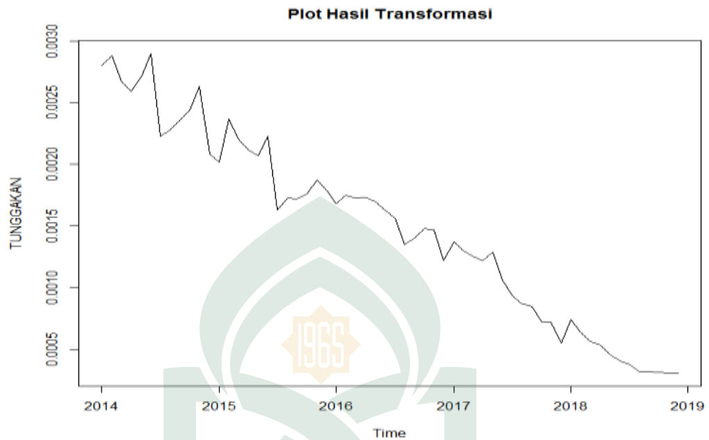
Gambar 4.6 Plot data setelah transformasi
