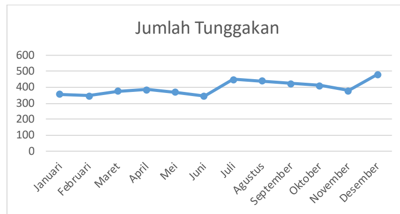
Gambar 4.2 grafik jumlah pemilik kendaraan tahun 2014
