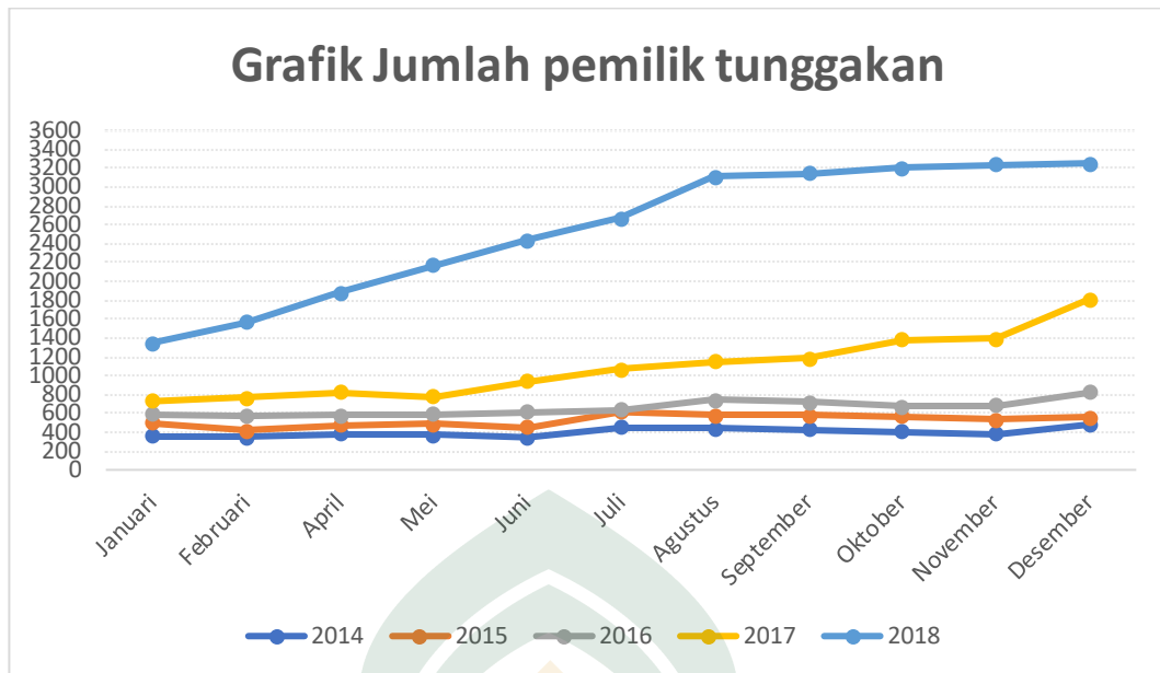
Gambar 4.1 Grafik Jumlah pemilik kendaraan menunggak 2014 -2018
