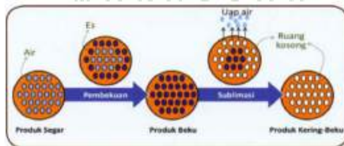
Gambar 11. Mekanisme pengeringan beku
