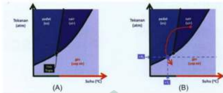
Gambar 12. Diagram Fase air
