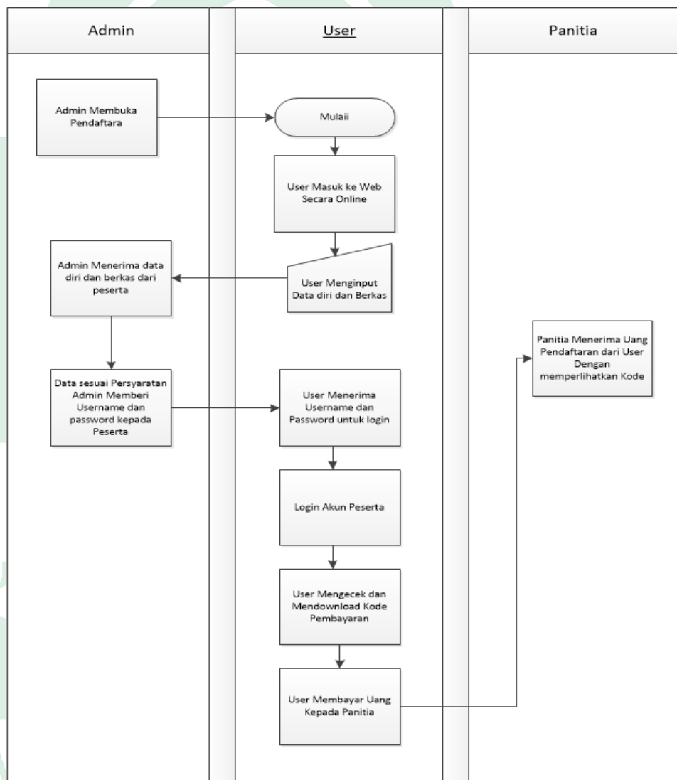
Gambar IV. 2 Flowmap Sistem yang sedang Diusulkan
