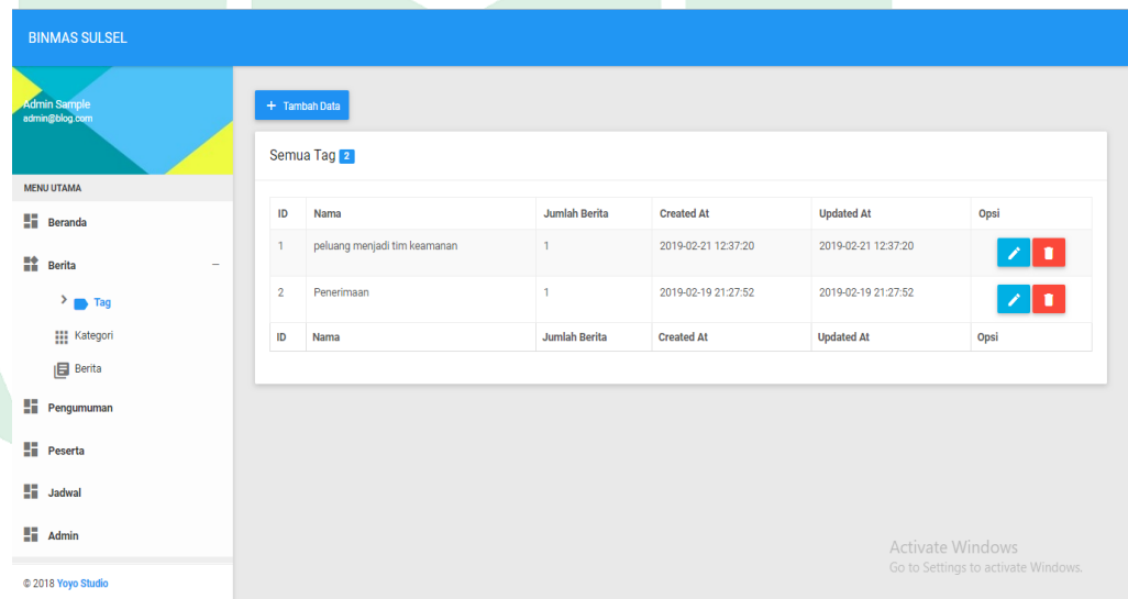
Gambar V. 3. Antarmuka Berita
