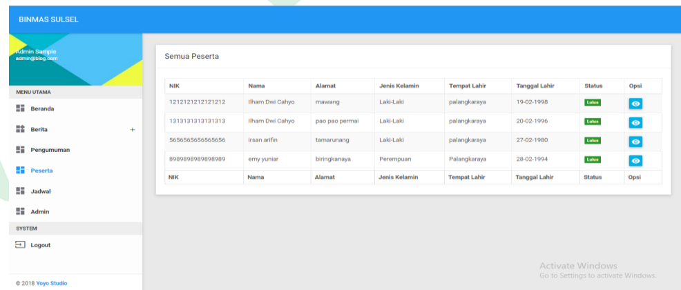
Gambar V. 5. Antarmuka peserta
