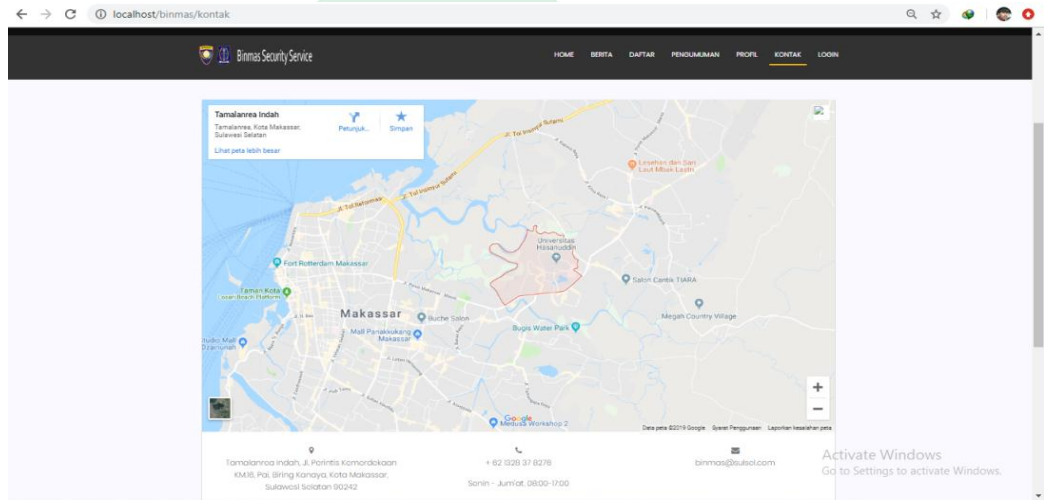
Gambar V. 12. Antarmuka kontak
