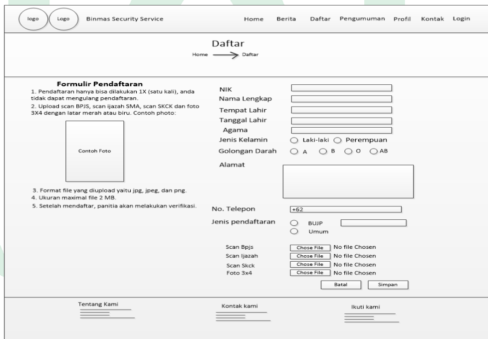
Gambar IV.11 rancangan pendaftaran
