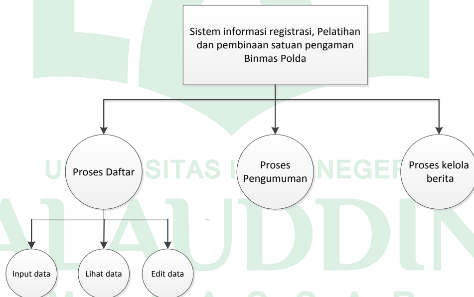
Gambar IV.4 Diagram HIPO
