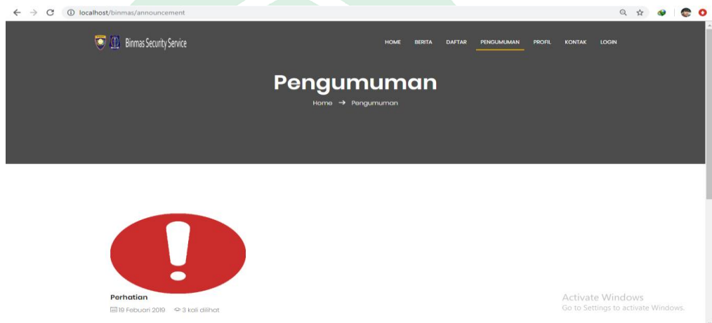
Gambar V. 10. Antarmuka Pengumuman
