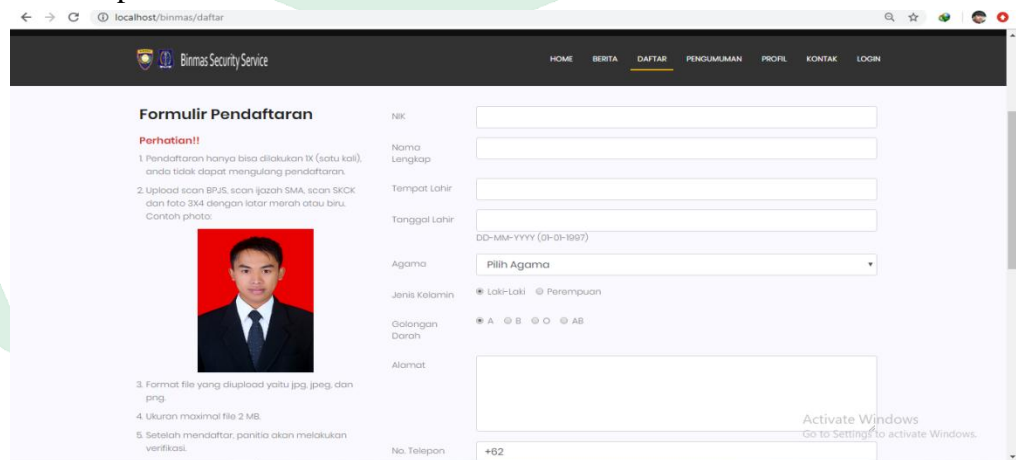
Gambar V. 9. Antarmuka Daftar
