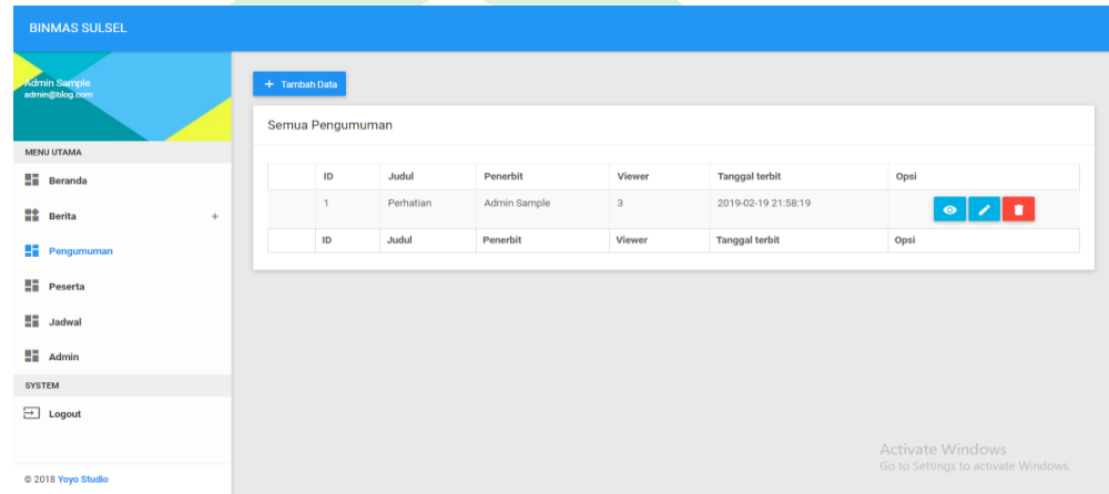
Gambar V. 4. Antarmuka pengumuman
