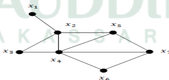
Gambar 2.19. Graph menggunakan algoritma Sequential Coloring .
