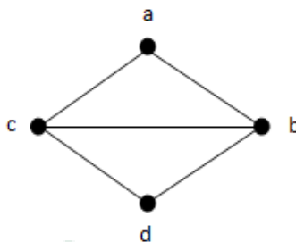
Gambar 2.9. Graph Sederhana.
