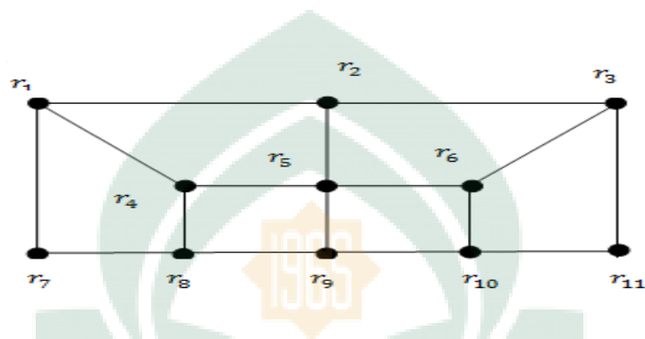
Gambar 2.18. Pemetaan P.
