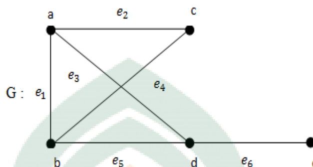
Gambar 2.4. Graph G Sederhana.
