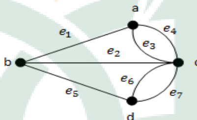
Gambar 2.10. Graph tak sederhana.
