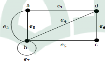
Gamabar 2.12. Graph tak berarah.
