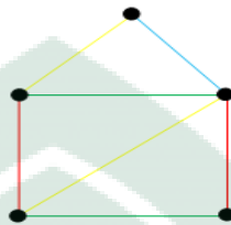
Gambar 2.15. Pewarnaan Sisi.
