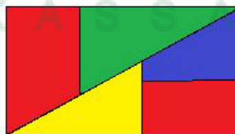
Gambar 2.16. Pewarnaan Wilayah.
