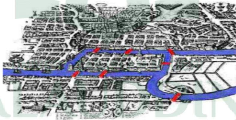
Gambar 2.1. Jembatan Königsberg. 4
