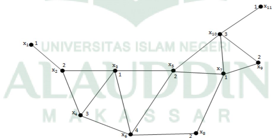
Gambar 4.6 : Graph yang Telah Diberi Warna (titik).
