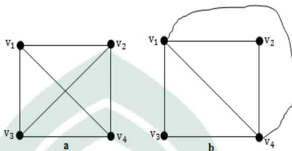
Gambar 2.13. Graph Planar dan Graph Bidang.
