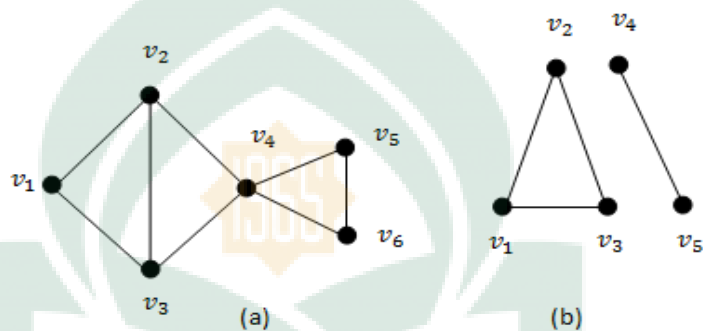
Gambar 2.8. Graph Terhubung dan Graph Tidak terhubung.
