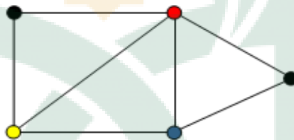
Gambar 2.14. Pewarnaan simpul.
