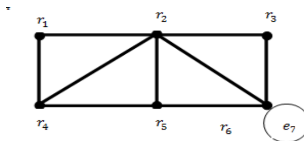
Gambar 2.17. Pemetaan M.
