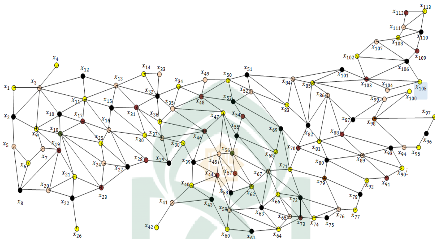
Gambar 4.7 : Graph Desa yang Telah Diberi Warna
