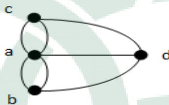
Gambar 2.2. Graph yang merepresentasikan jembatan konigsberg.
