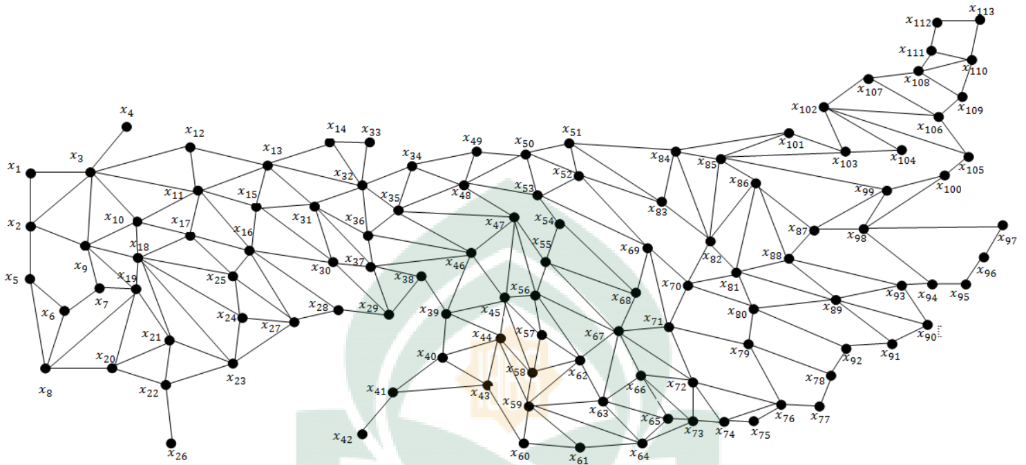
Gambar 4.5 : Graph Kab. Jeneponto Berdasarkan Wilayah Desa.
