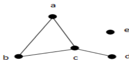
Gambar 2.6. Simpul Terpencil.
