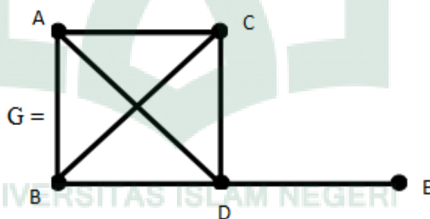
Gambar 2.3. Graph G Sederhana.
