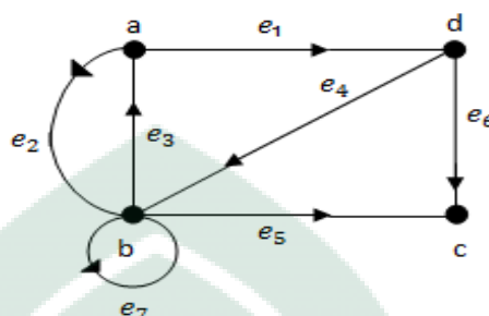
Gamabar 2.11. Graph berarah.
