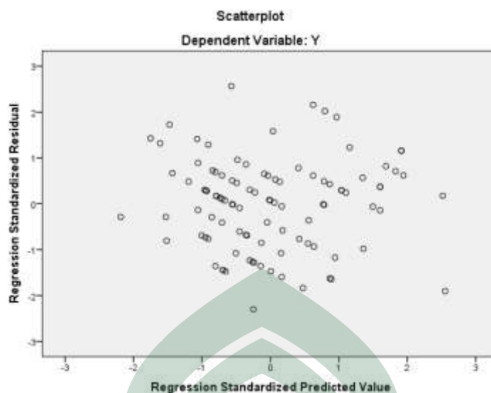
Gambar 4.3 Grafik Scatterplot
