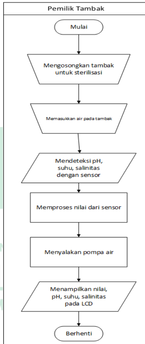
Gambar IV.8 Flowmap Diagram Analisis Sistem yang diusulkan.
