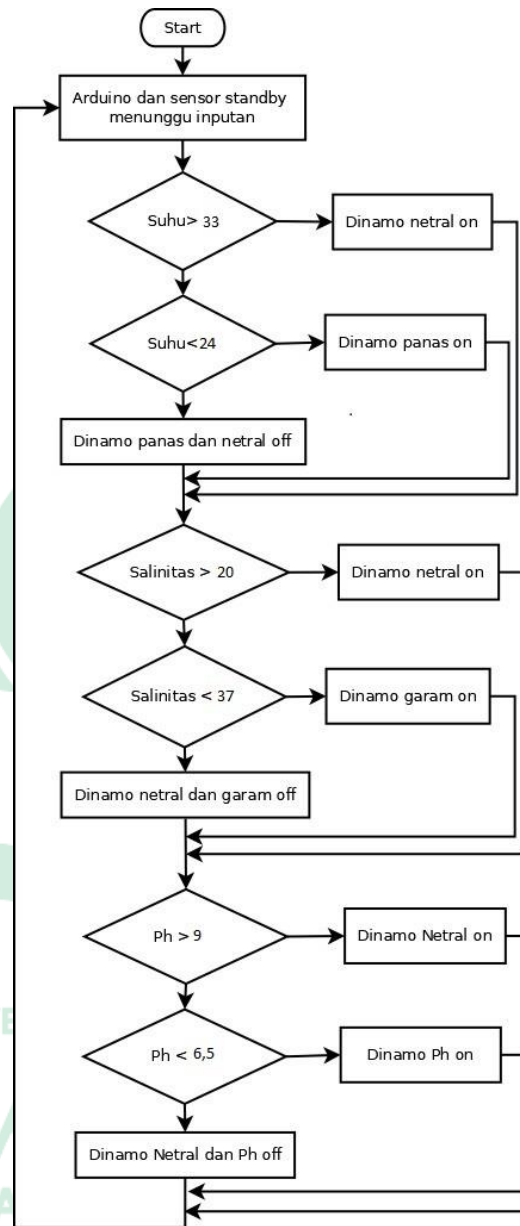
Gambar IV.10. Rangkaian Flowchart Sistem Alat Pengendali pH, Suhu Dan Salinitas Air Pada Tambak Berbasis Mikrokontroler.
