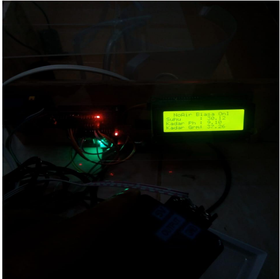
Gambar V.25 Pengujian sensor salinitas dengan kadar garam di atas standar
