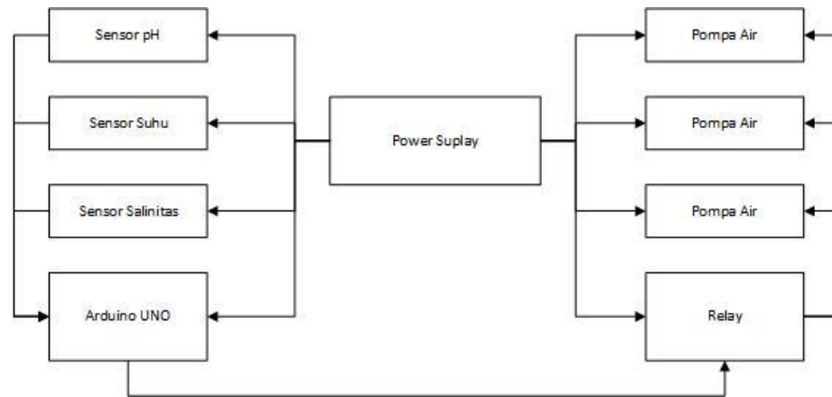
Gambar IV.9. Diagram Blok alat pengendali pH, suhu dan salinitas air pada tambak berbasis mikrokontroler terdiri dari beberapa masukan dan keluaran.
