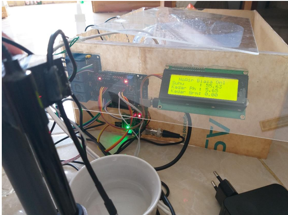
Gambar V.21 Pengujian sensor suhu dengan suhu di atas normal
