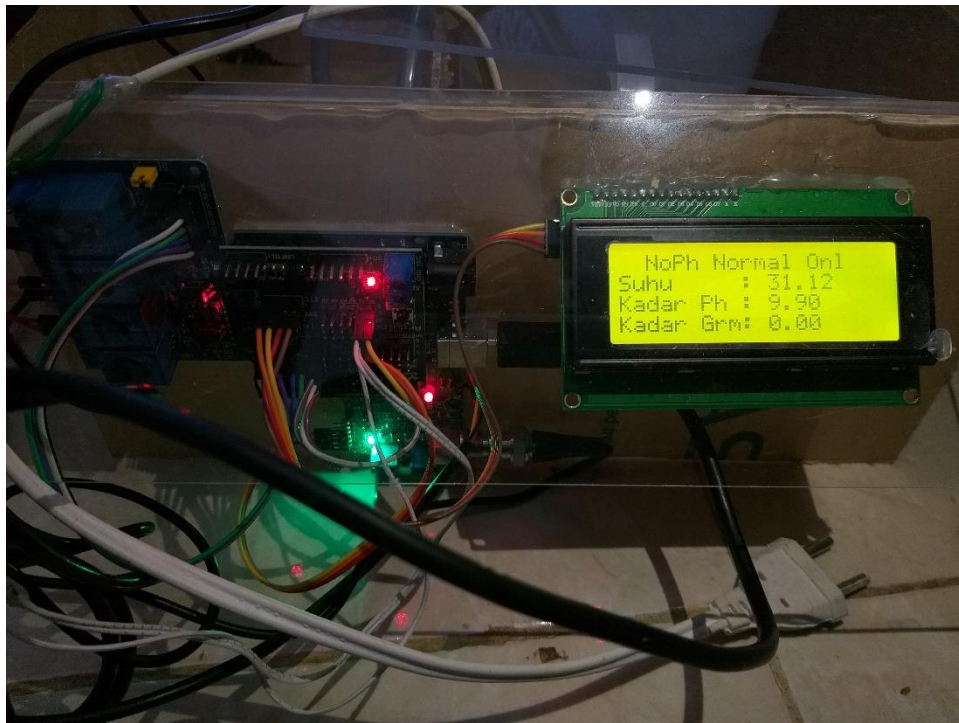
Gambar V.19 Pengujian sensor Ph di atas nilai standar
