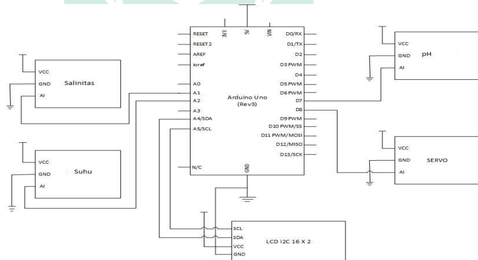
Gambar IV.12. Rancangan Keseluruhan Sistem 2D
