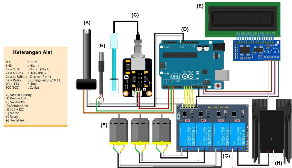
Gambar IV.11. Rancangan Keseluruhan Sistem
