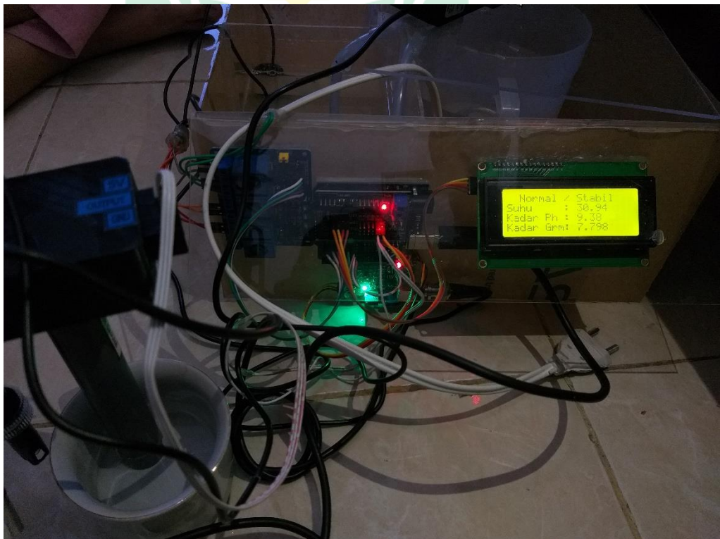
Gambar V.23 Pengujian sensor salinitas dengan kadar garam di bawah standar
