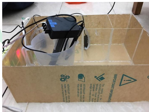
Gambar V.13 Tampak sisi kiri dan kanan alat
