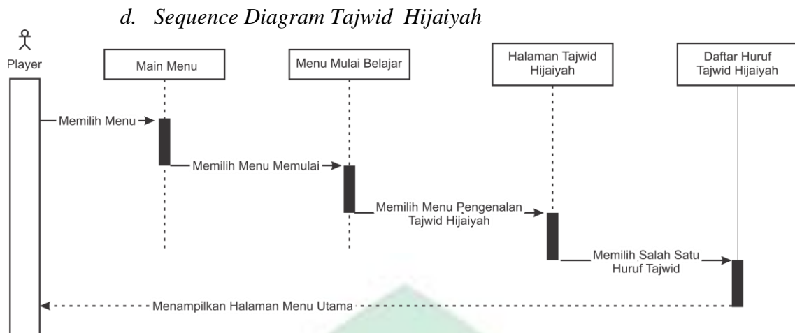
Gambar IV.12. Sequence Diagram Tajwid Hijaiyah
