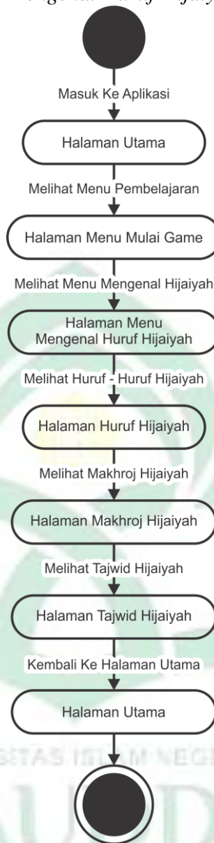
Gambar IV.4. Statechart Diagram Mengenal Huruf Hijaiyah
