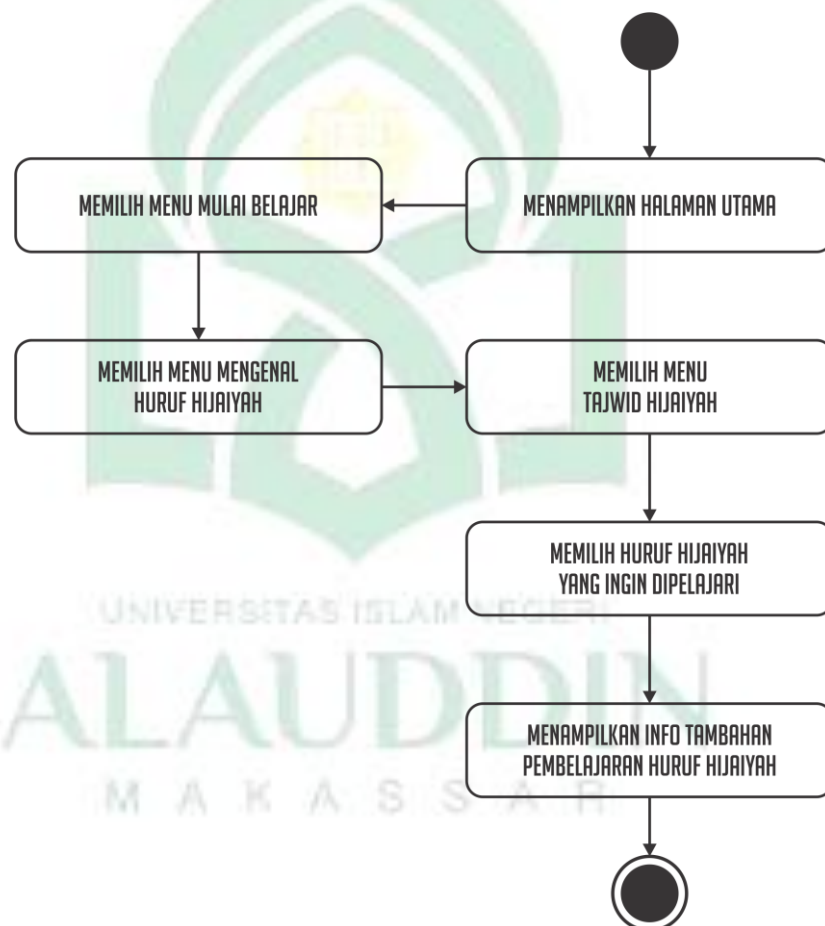
Gambar IV.6. Activity Diagram Mengenal Tajwid Hijaiyah
