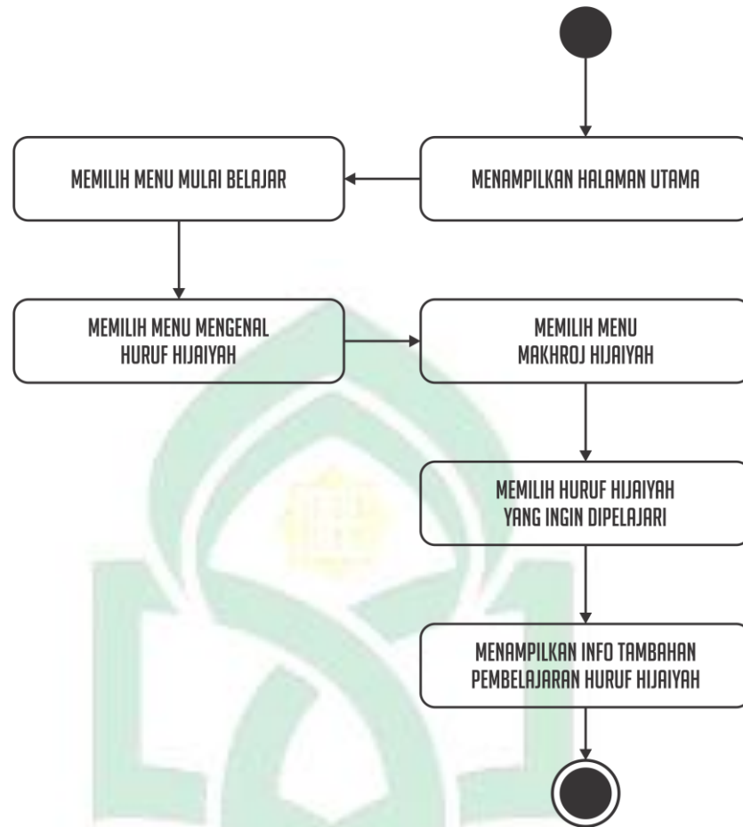
Gambar IV.5. Activity Diagram Mengenal Makhroj Hijaiyah
