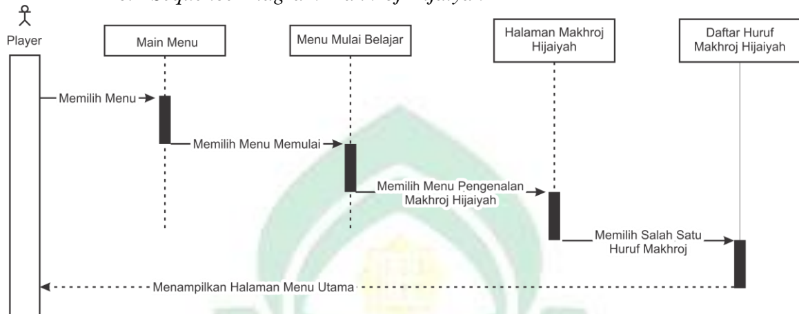
Gambar IV.11. Sequence Diagram Makhroj Hijaiyah
