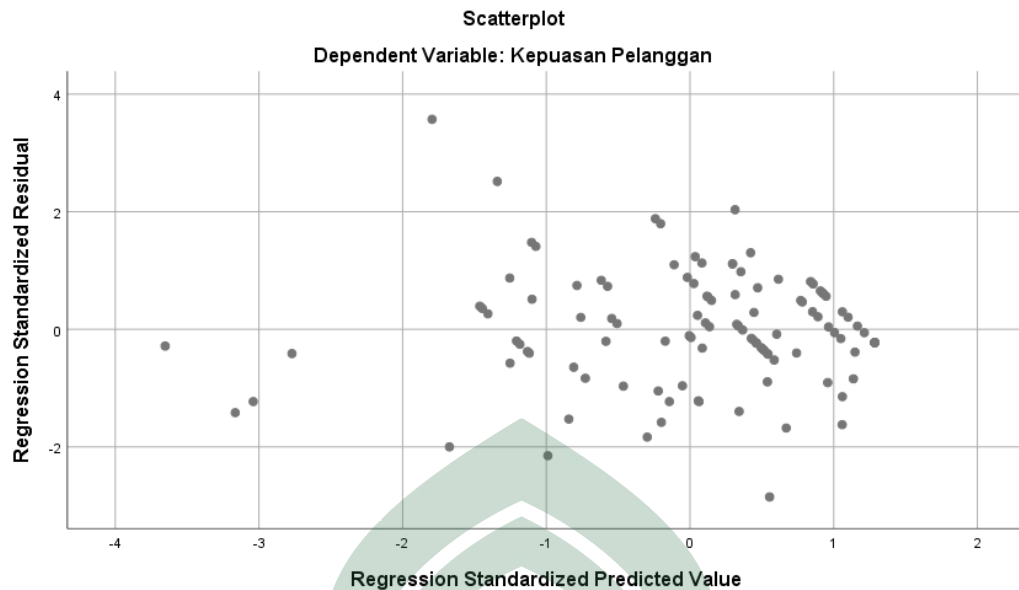
Gambar 4.2 Uji Heteroskedastisitas
