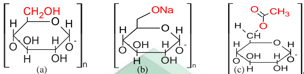
Gambar 4. 2 Perbedaan struktur (a), pati biji nangka ( Artocarpus heterophyllus L.) (b), pati biji nangka teraktivasi NaOH (c) pati biji nangka termodifikasi asetat
