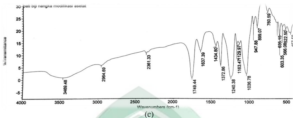
Gambar 4.1 Hasil FTIR (a) Pati biji nangka ( Artocarpus heterophyllus L.), (b) Pati biji nangka teraktivasi NaOH (c), Pati asetat biji nangka ( Artocarpus heterophyllus L.)
