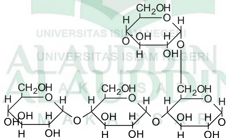
Gambar 2. 3 Amilopektin (Poedjiadi dan Titin, 2007)
