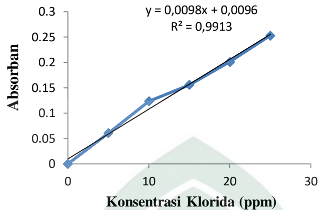
Gambar 4. 4 Grafik Kurva Standar Klorida
