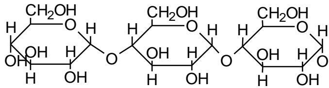
Gambar 2. 2 Amilosa (Poedjiadi dan Titin, 2007)
