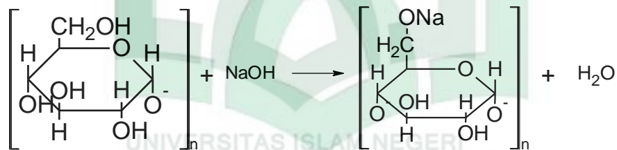
Gambar 4. 6 Reaksi pati biji nangka dengan NaOH (Sangsheethong, dkk., 2005)
