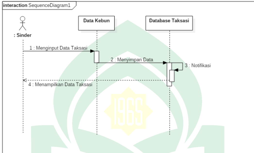
Gambar IV. 7 Sequence Diagram untuk Menu Sinder Kebun Wilayah
