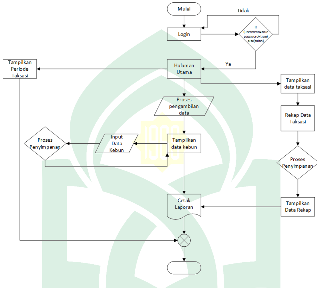
Gambar IV. 8 Flowchart untuk Admin
