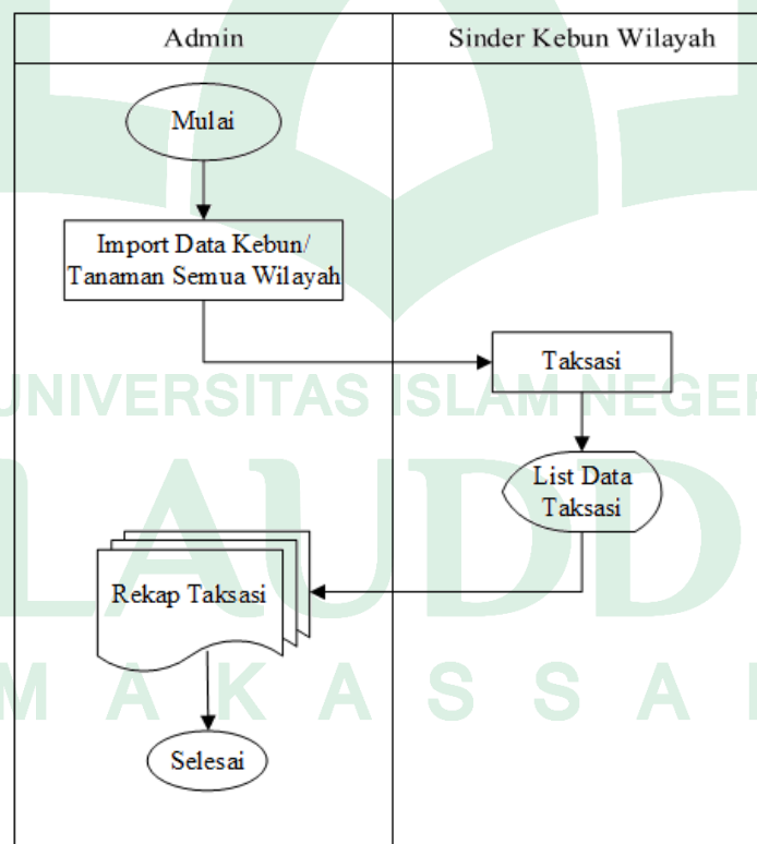
Gambar IV. 2 Flowmap sistem yang diusulkan
