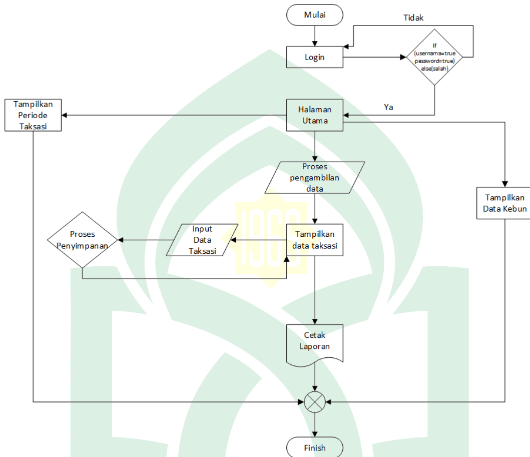
Gambar IV. 9 Flowchart untuk Sinder Kebun Wilayah
