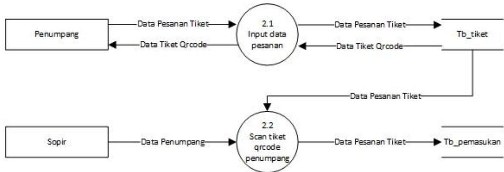
Gambar IV.8 Diagram level 2 proses 2 (proses pembayaran dan validasi)
