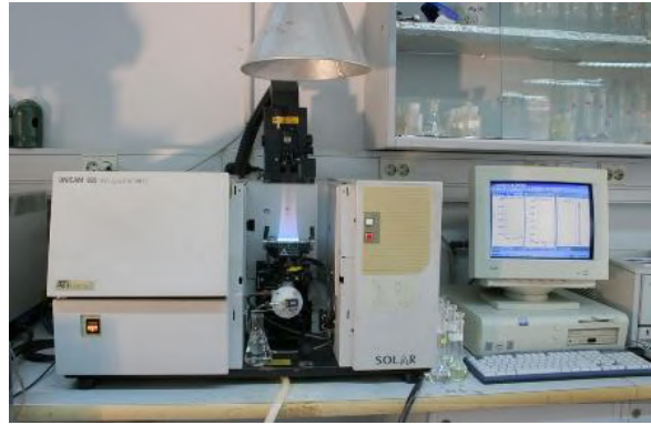
Gambar 2.4 Spektrofotometri Serapan Atom (SSA) (UIN Alauddin Makassar).
