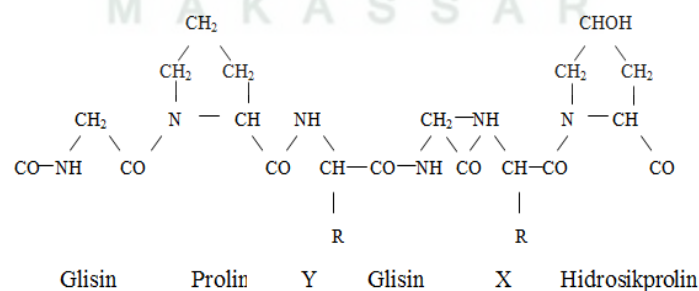
Gambar 2.2 Struktur Kimia Gelatin (Grobben dkk, 2004 dalam Ramadani, 2014:22)
