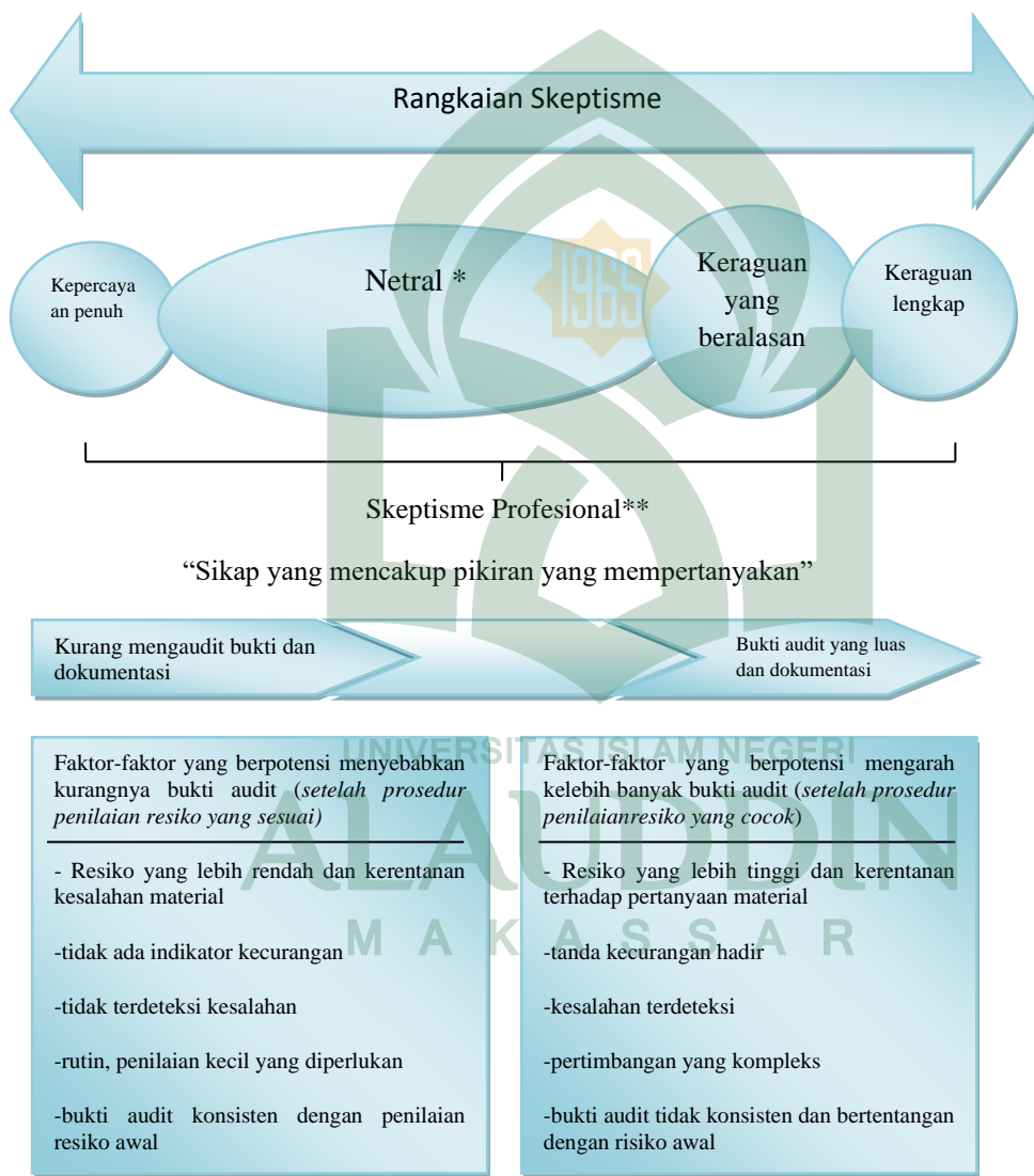
Gambar 2.1 Rangkaian Skeptisme
