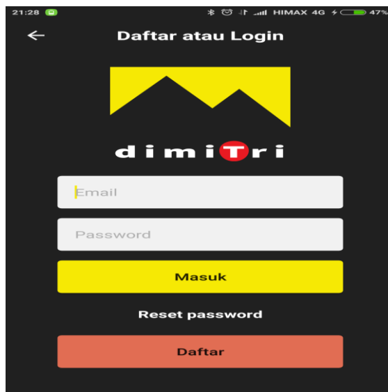
Gambar V .1. Antarmuka login
