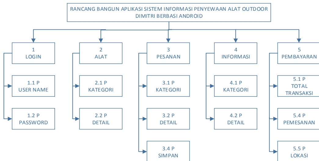
Gambar IV .12. Diagram Berjenjang
