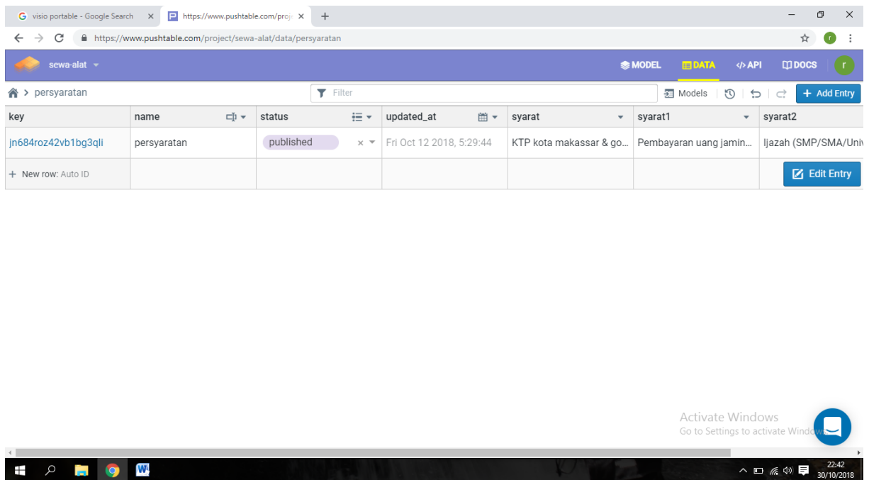
Gambar. V.19. Halaman Persyaratan
