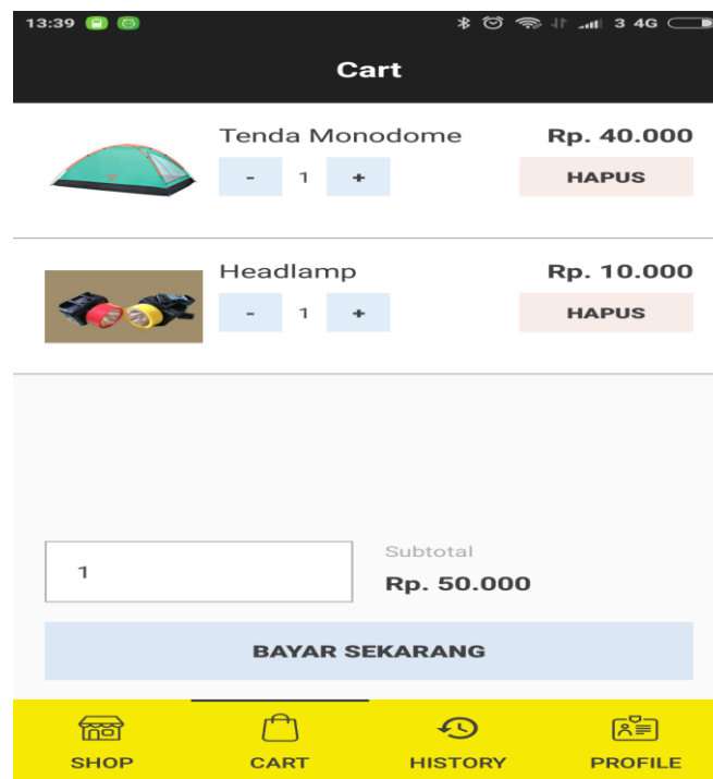
Gambar V. 5. Menu pemesanan
