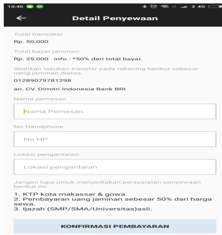
Gambar V.6. Detail penyewaan
