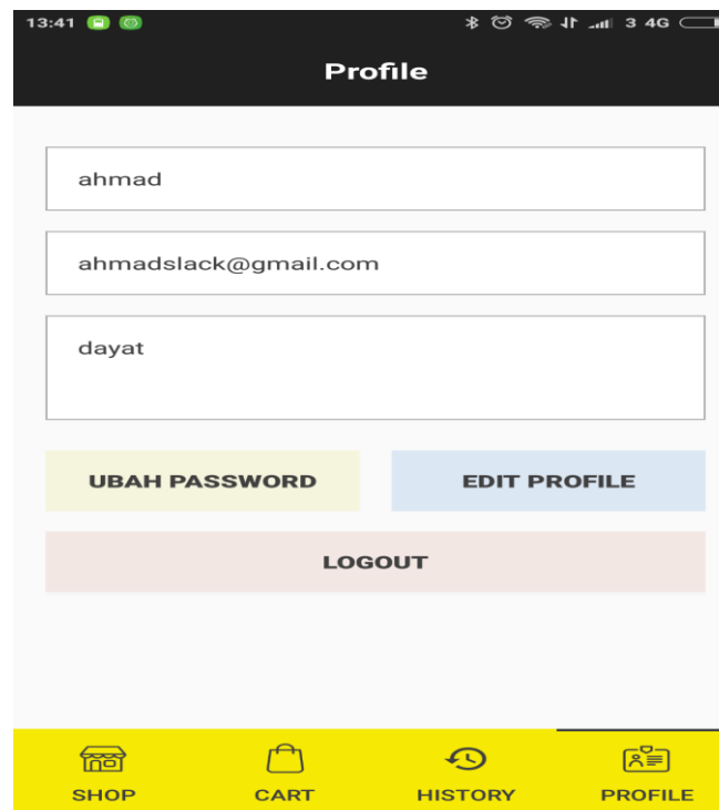
Gambar V .10. Antarmuka Profile
