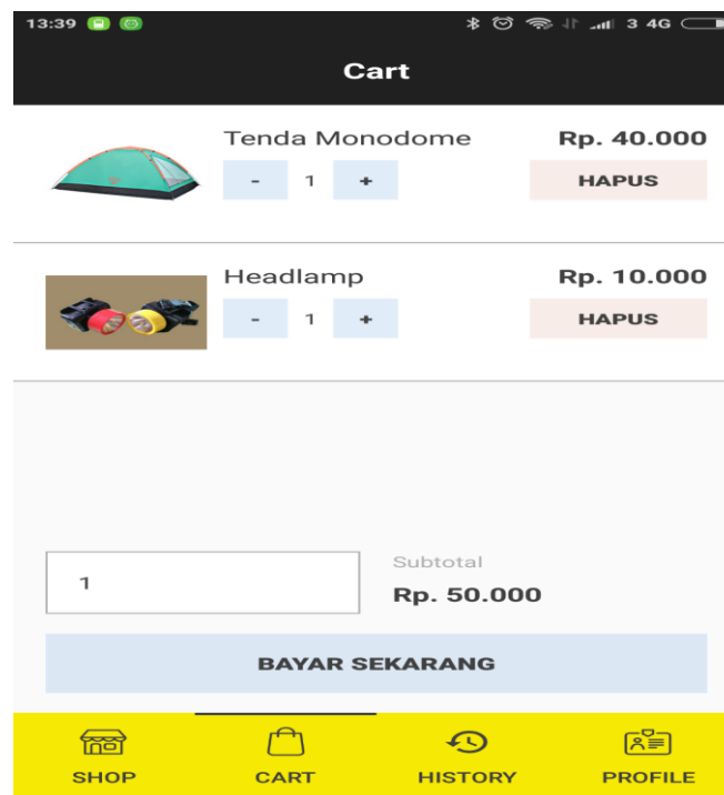
Gambar V .4. Menu Cart
