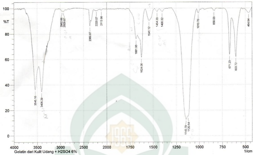
Gambar 4.9. Analisis FTIR Gelatin Kulit Udang Jerbung + H 2 SO 4 6%
