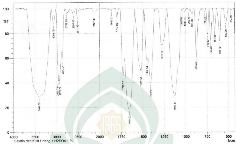
Gambar 4.7. Analisis FTIR Gelatin Kulit Udang Jerbung + H 2 SO 4 1%
