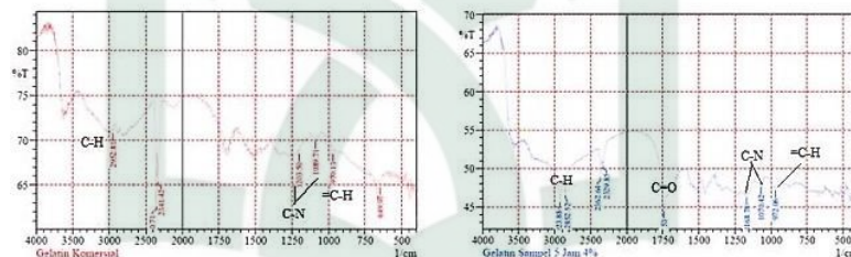
Gambar 2.5 Analisis FTIR Gelatin Komersial dan Gelatin Tulang Ikan Lele (Sumber: Permata, dkk., 2016: 149)
