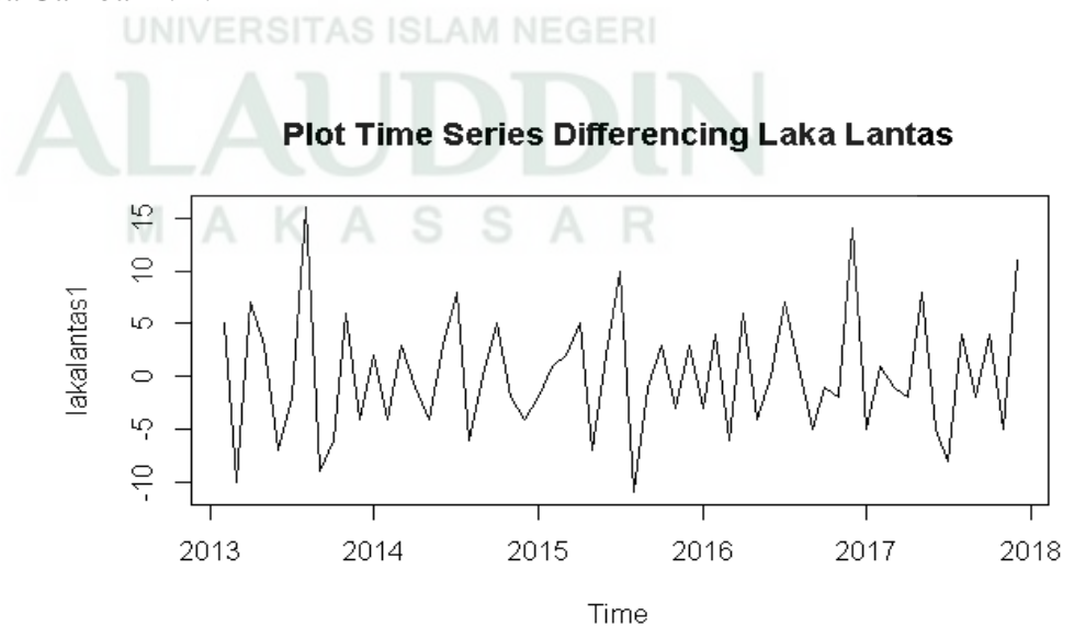
Gambar 4.2 Differencing Jumlah Laka Lantas
