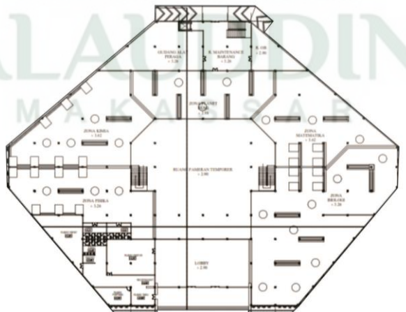
Gambar V.5 Transformasi Akhir Lantai 1 Bangunan Utama (Sumber : Hasil Desain, 2019)
