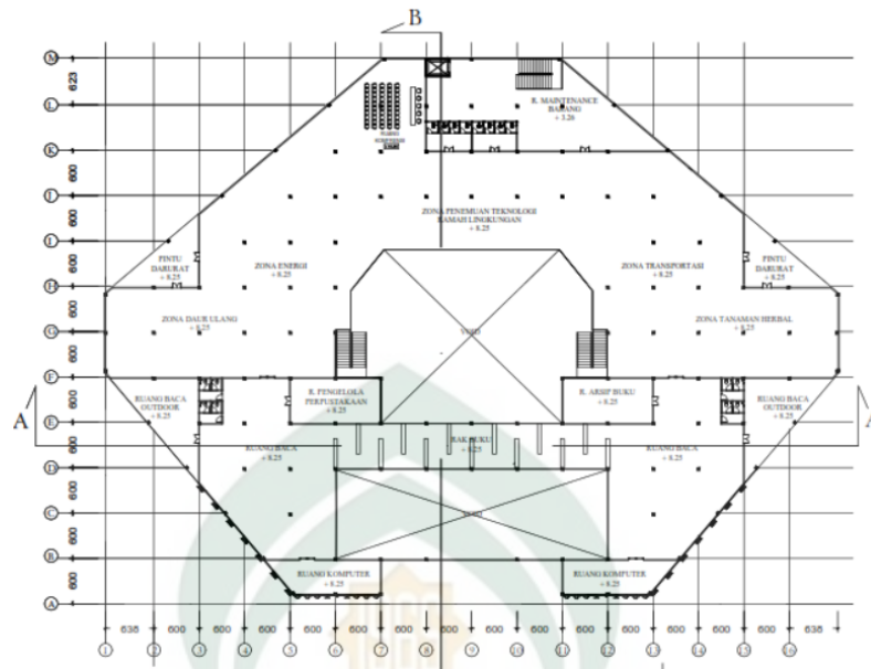
Gambar VI.3 Tampilan Denah Lantai 1 (Sumber : Hasil Desain, 2019)
