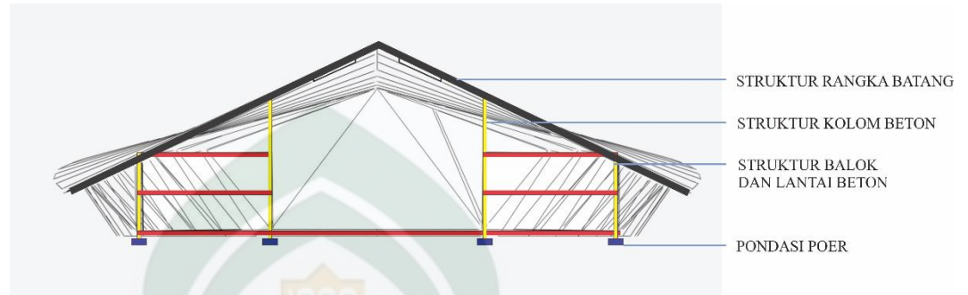
Gambar IV.13 Struktur Bangunan Sumber : Olah Desain, 2018
