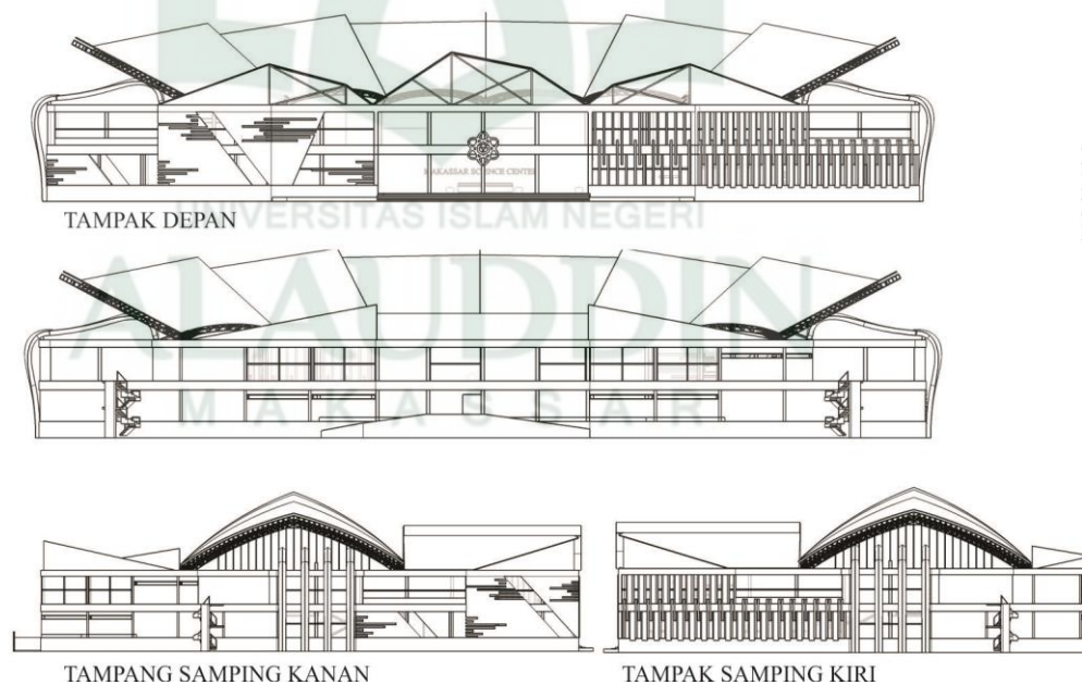
Gambar V.9 Transformasi Akhir Bangunan Utama (Sumber : Hasil Desain, 2019)
