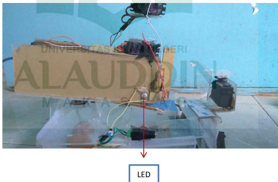
Gambar V. 2 Sistem penyortiran kualitas telur ayam ras berbasis mikrokontroler (tampak samping kanan)
