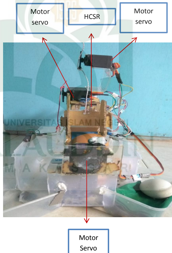
Gambar V. 1 Sistem penyortir kualitas telur ayam ras berbasis mikrokontroler (tampak depan)
