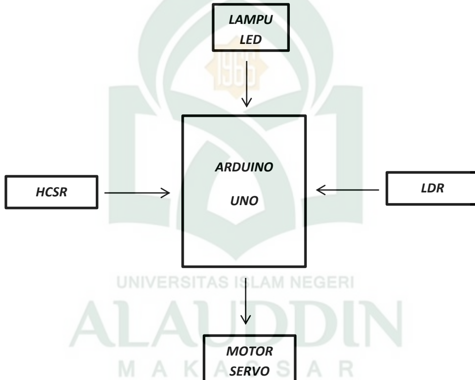
Gambar IV. 1 Diagram Blok Sistem Alat
