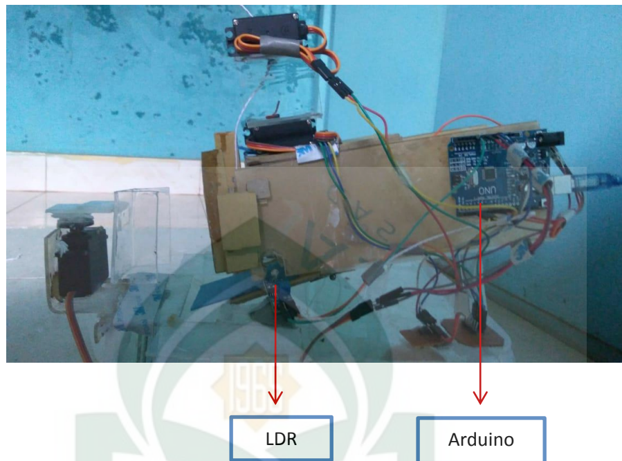
Gambar V. 2 Sistem penyortiran kualitas telur ayam ras berbasis mikrokontroler (tampak samping kanan)
