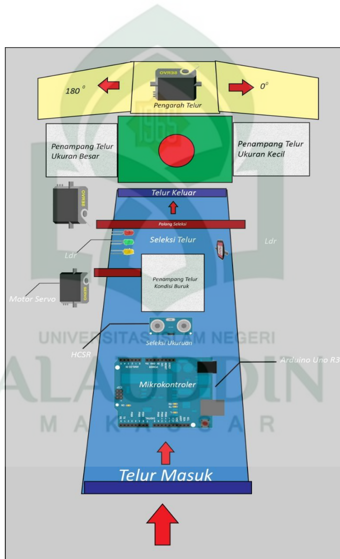
Gambar IV. 3 Rancangan Keseluruhan Alat
