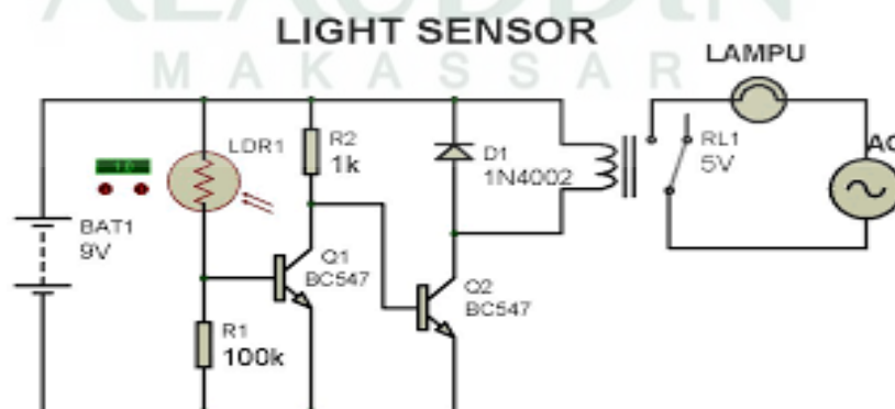
Gambar IV. 9 Rangkaian LDR
