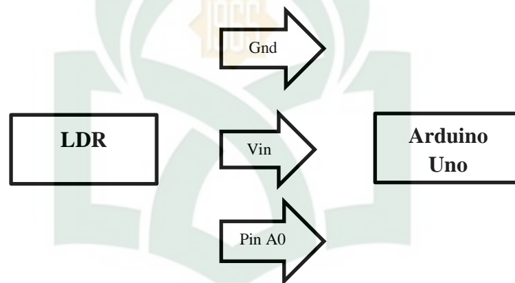
Gambar IV. 8 Ilustrasi pin sensor LDR
