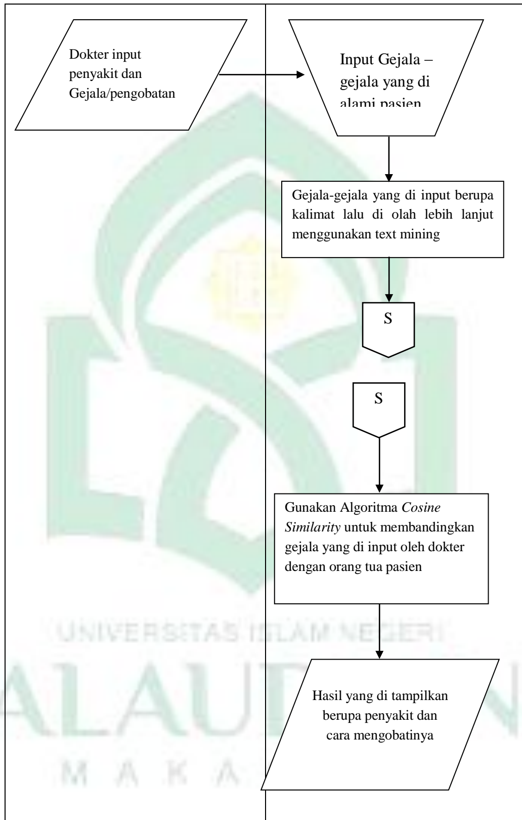
Gambar IV.2 Flowmap sistem yang diusulkan
