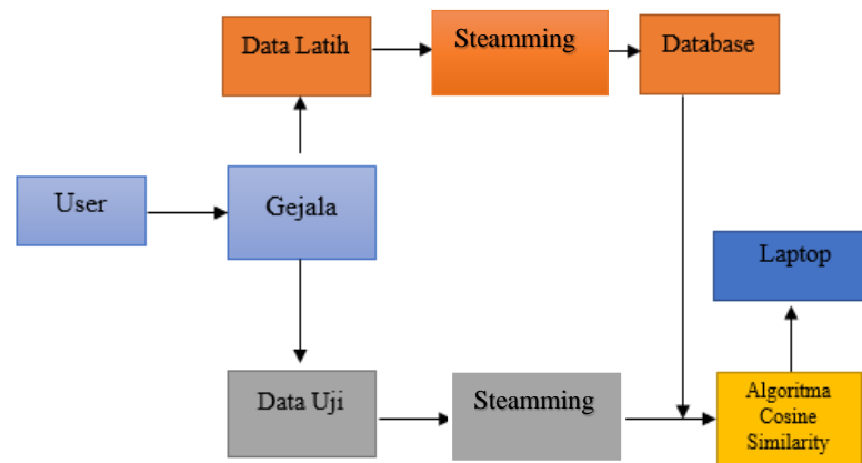
Gambar IV.3 Bagan Diagram Blok
