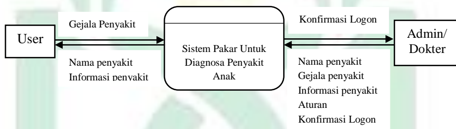
Gambar IV.10 Diagram Konteks
