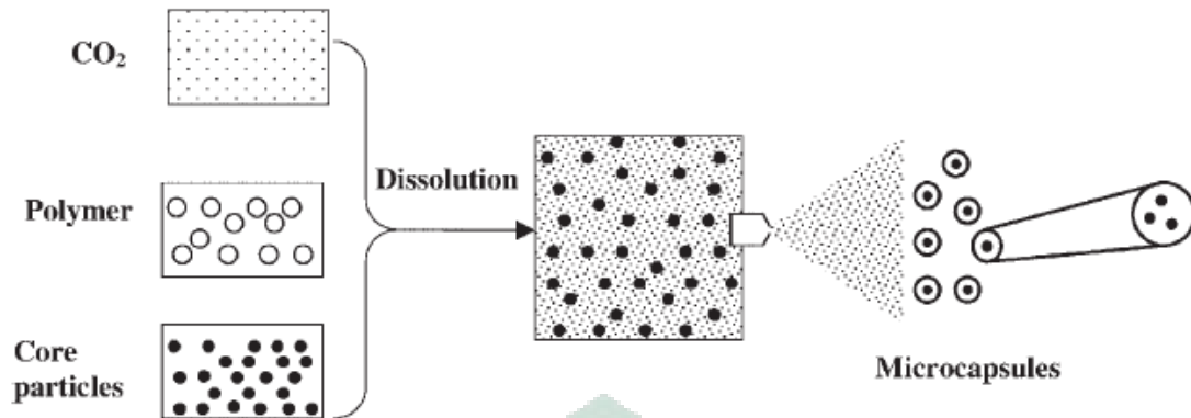
Gambar 4. Mikroenkapsulasi dengan ekspansi cepat dari cairan superkritis
