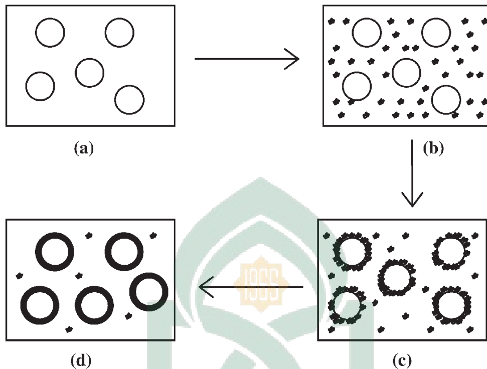
Gambar 3. Proses Koaservasi: (a) Dispersi bahan inti dalam larutan polimer (b) Pemisahan koaservat dari larutan (c) Pelapisan bahan inti oleh tetesan mikro koaservat (d) Koalesensi koaservat untuk membentuk cangkang kontinyu disekitar partikel.
