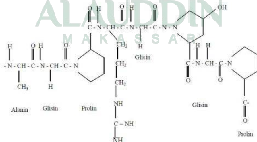
Gambar 7. Struktur Kimia Gelatin (Chaplin, 2006)
