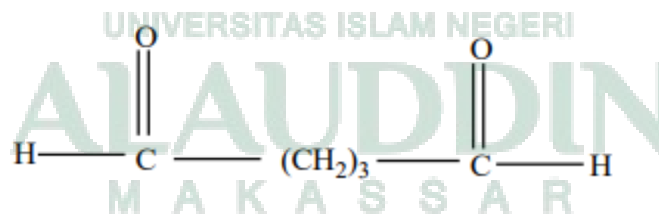
Gambar 9. Struktur Glutaraldehyd
