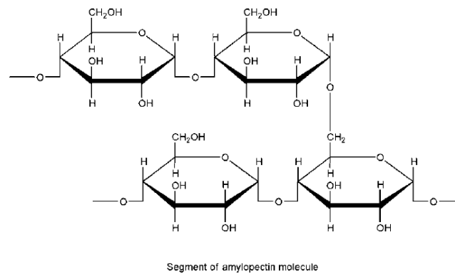
Gambar 3 : Amilopektin
