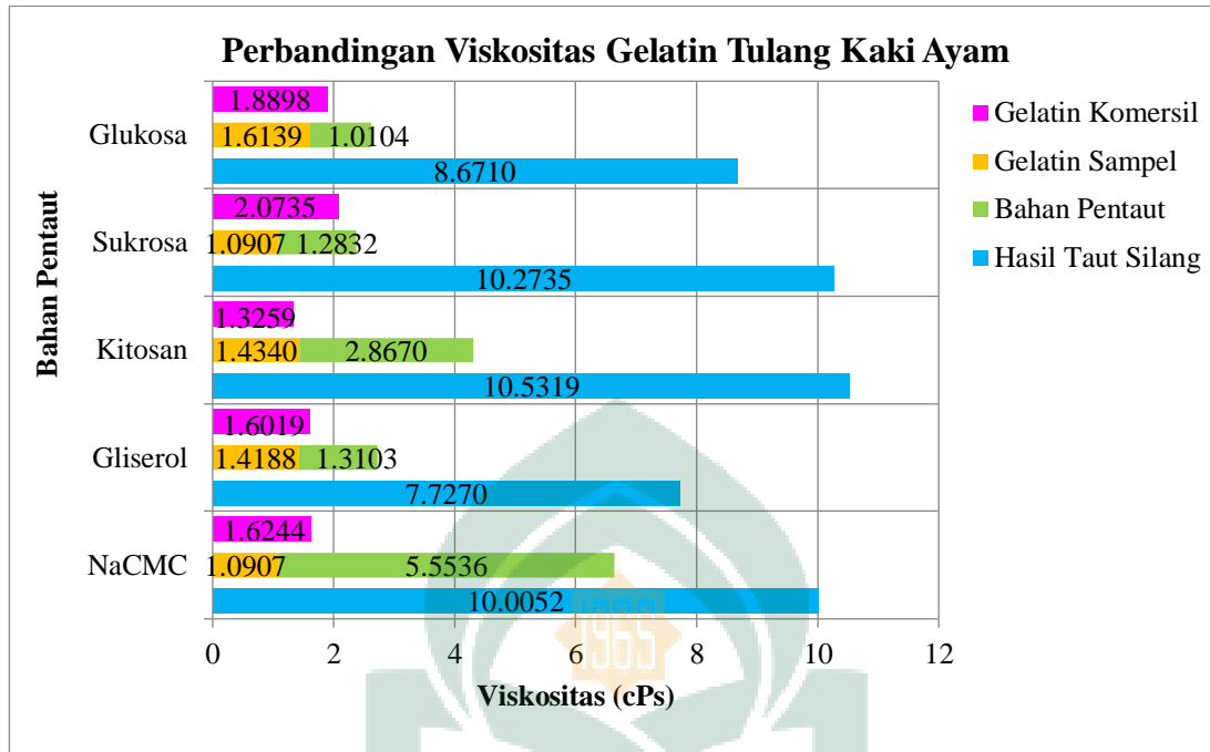
Gambar 22. Histogram Perbandingan Uji Viskositas Gelatin Tulang Kaki Ayam
