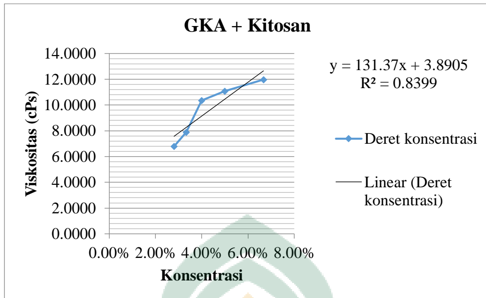
Gambar 28. Grafik Uji Viskositas Gelatin Kulit Ayam Taut Silang Kitosan
