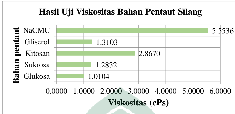
Gambar 19. Histogram Pengujian Viskositas Bahan Pentaut Silang
