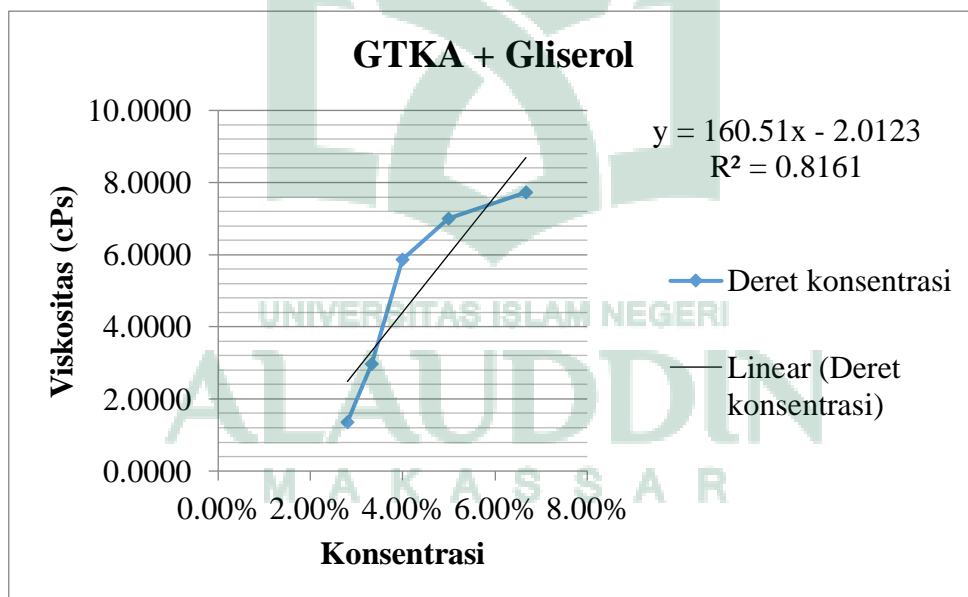
Gambar 31. Grafik Uji Viskositas Gelatin Tulang Kaki Ayam Taut Silang Gliserol
