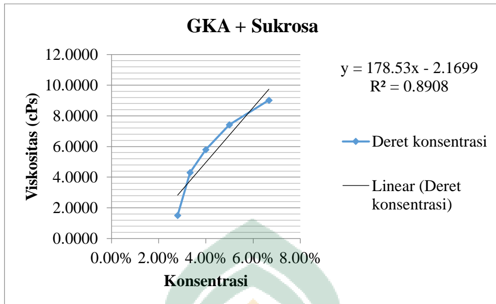
Gambar 26. Grafik Uji Viskositas Gelatin Kulit Ayam Taut Silang Sukrosa
