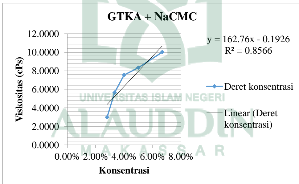
Gambar 33. Grafik Uji Viskositas Gelatin Tulang Kaki Ayam Taut Silang NaCMC
