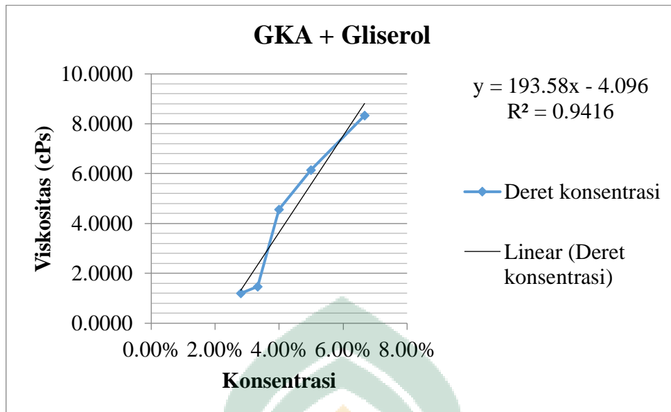
Gambar 30. Grafik Uji Viskositas Gelatin Kulit Ayam Taut Silang Gliserol
