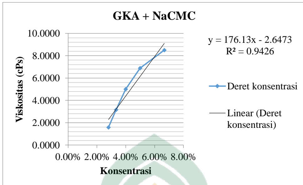
Gambar 32. Grafik Uji Viskositas Gelatin Kulit Ayam Taut Silang NaCMC
