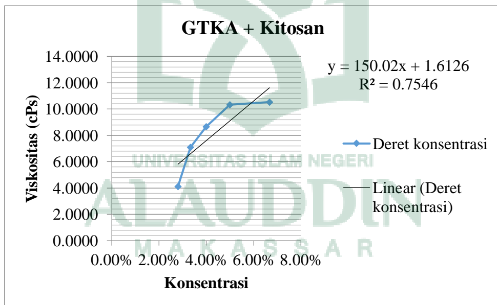
Gambar 29. Grafik Uji Viskositas Gelatin Tulang Kaki Ayam Taut Silang Kitosan
