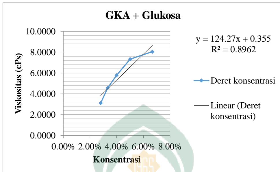
Gambar 24. Grafik Uji Viskositas Gelatin Kulit Ayam Taut Silang Glukosa
