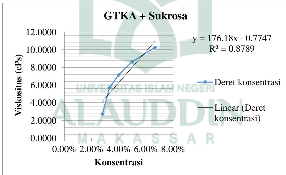
Gambar 27. Grafik Uji Viskositas Gelatin Tulang Kaki Ayam Taut Silang Sukrosa
