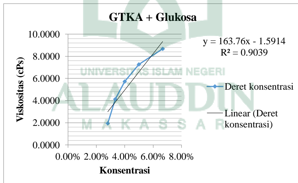
Gambar 25. Grafik Uji Viskositas Gelatin Tulang Kaki Ayam Taut Silang Glukosa
