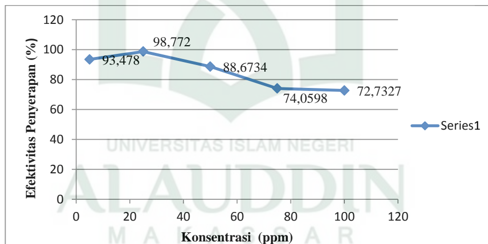
Gambar IV. 6 Grafik hubungan antara konsentrasi dengan efektivitas penyerapan
