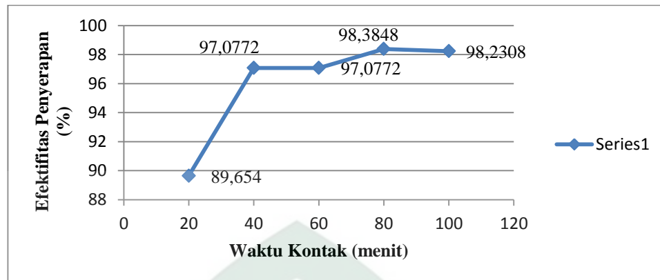
Gambar IV. 7 grafik hubungan antara waktu kontak dengan efektivitas penyerapan
