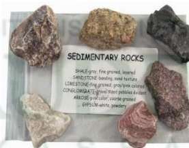
Gambar II. 2 Batuan Sedimen
