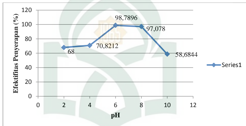
Gambar IV. 8 grafik hubungan antara pH dengan efektivitas penyerapan
