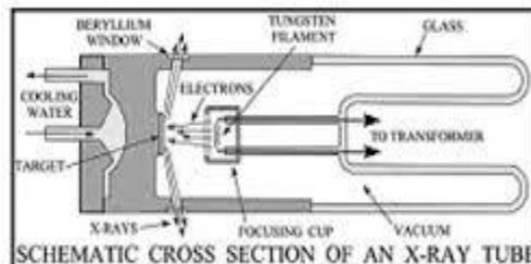
Gambar II. 4 Skema Tabung Sinar x
